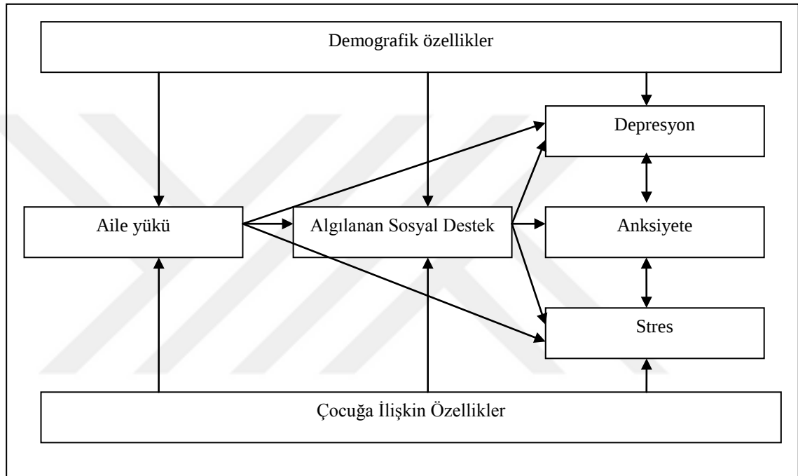
Şekil 1.1: Hipotez Şeması
