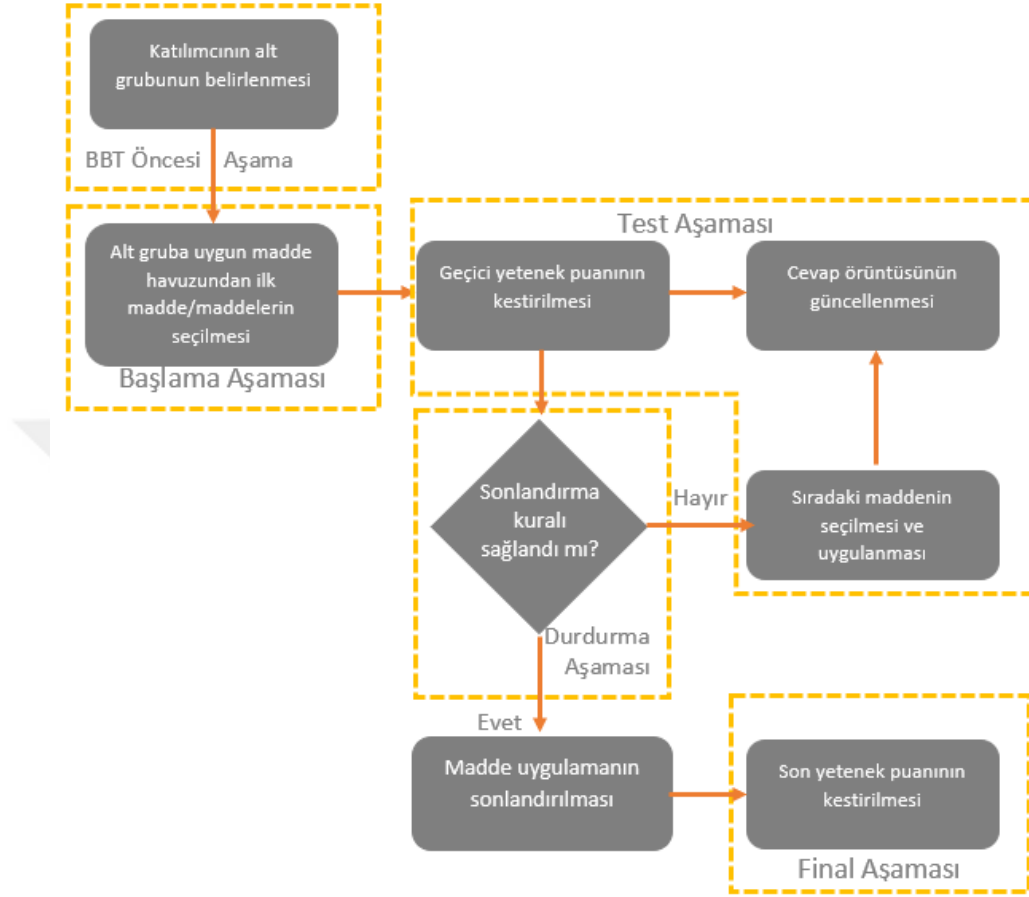
Şekil 4. AMTM için BBT post-hoc simülasyon şeması
