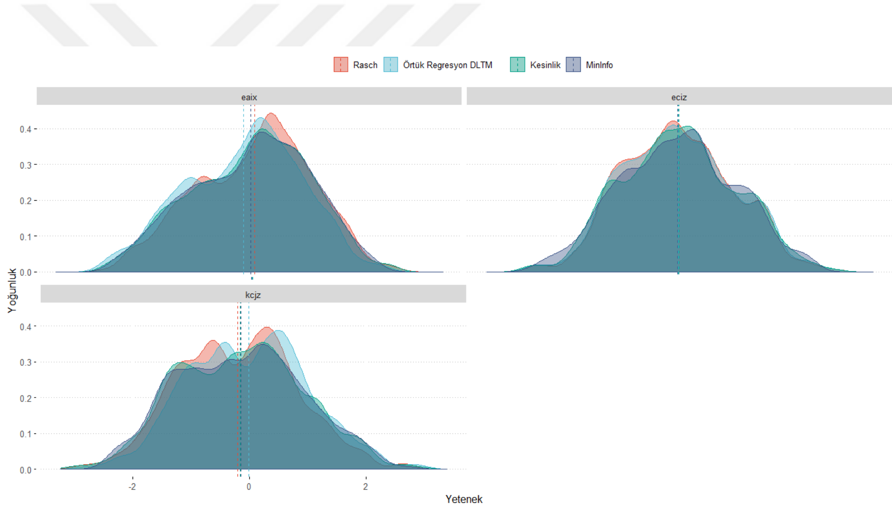
Şekil 20. ÖRDLTM parametrelerine dayalı BBT simülasyonlarında kestirilen yetenek puanlarının dağılımı
