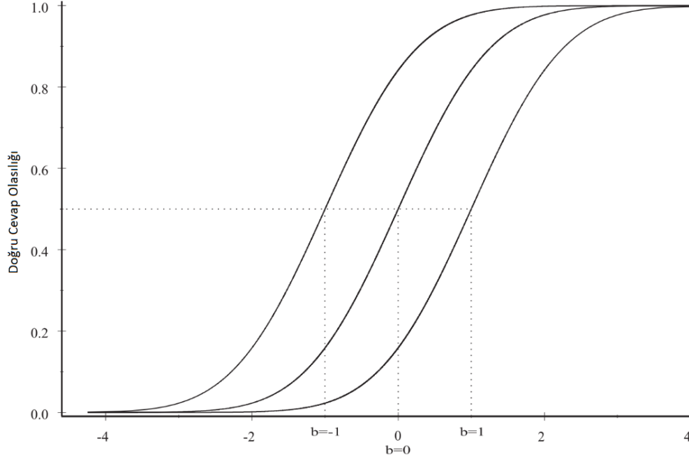
Şekil 1. Rasch modeline ilişkin madde karakteristik eğrisi
