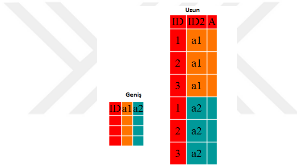
Şekil 3. Verilerin geniş ve uzun biçimleri
