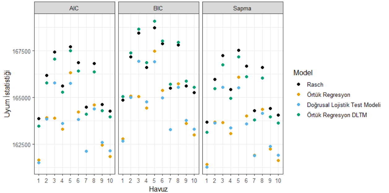
Şekil 11. Madde havuzu bazında model-veri uyum indeksleri
