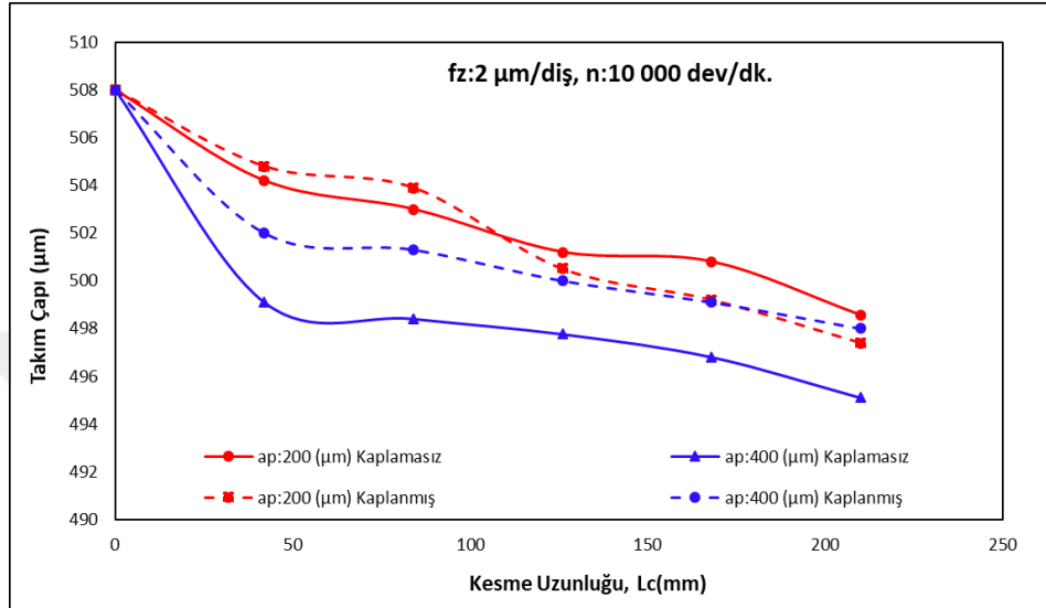
Şekil 4. 8 Kaplamasız ve elmas kaplanmış kesme uzunluęuna baęlı olarak farklı talaş derinlięi için elde edilen takım apındaki değışimin grafięi.
