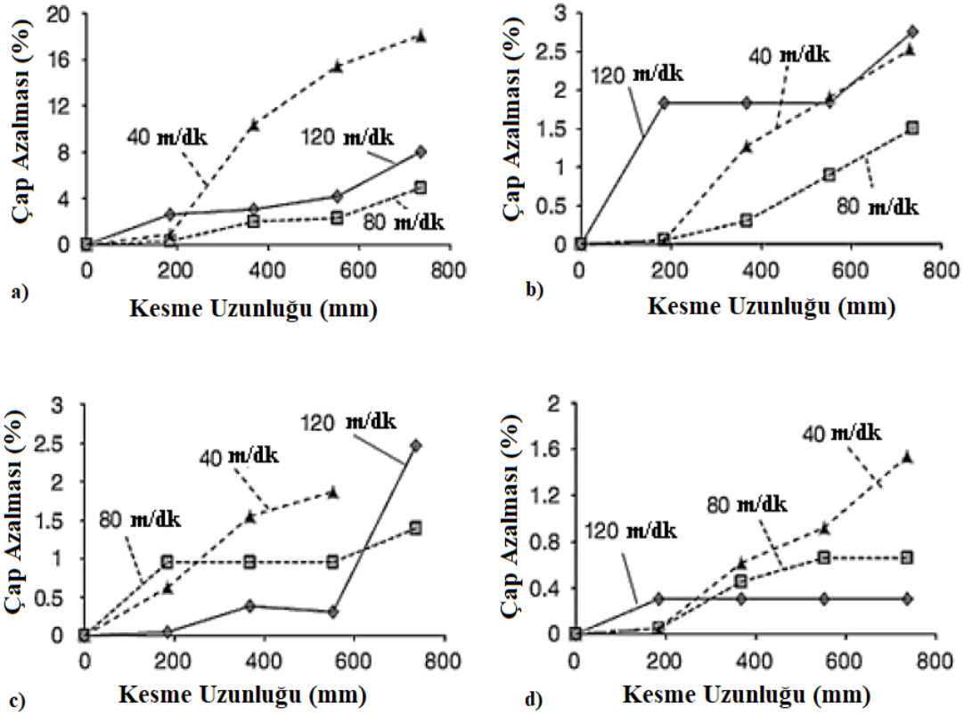
Şekil 2. 19 Fark ilerleme hızlarında aşınmaya bağlı olarak kesici takımda oluşan çap değişimi a) 0,75 µm/dk b) 1,5 µm/dk c) 3 µm/dk d) 6 µm/dk (Filiz et al. 2007).
