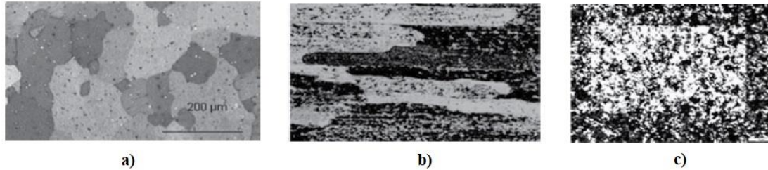
Şekil 2. 7 Al 5083’ün mikro yapıları: a) işlemden önce, b) konvansiyonel işleminden sonra, c) ECAP işleminden sonra (Popov et al. 2006).
