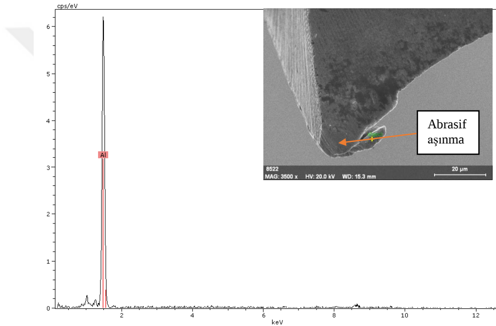
Şekil 4. 14 Kaplamasız takımın ( f_z=100 \mu\text{m}/\text{diş} , n=10\,000 \text{ dev}/\text{dk.} , a_p=200 \mu\text{m} ) kesme işlemi esnasında meydana gelen talaş yapışması ve EDX analizi görüntüleri.
