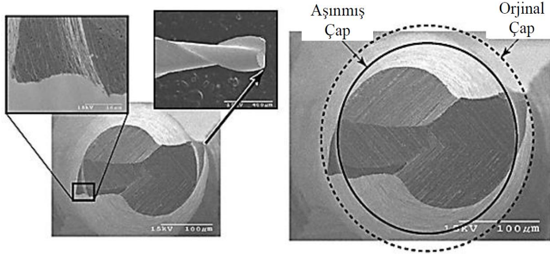
Şekil 2. 21 Mikro işlemede aşınmaya bağlı olarak kesici takım çapındaki değişimi (Filiz et al. 2007).
