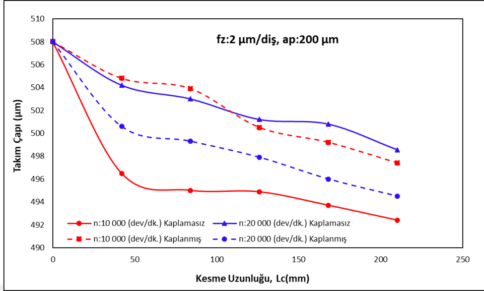
Şekil 4. 9 Kaplamsız ve elmas kaplanmış farklı devir sayıları için kesme uzunluğuna bağlı olarak takım çapında meydana gelen değişimi.
