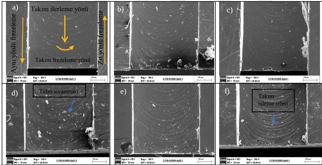
Şekil 4. 21 Kaplamasız ve elmas kaplanmış takımlar için farklı talaş derinliği değerleri için elde edilen işlenmiş kanal görüntüleri (sabitler; n=10\,000 dev/dk., fz=2 \mu\text{m}/\text{diş} ).
