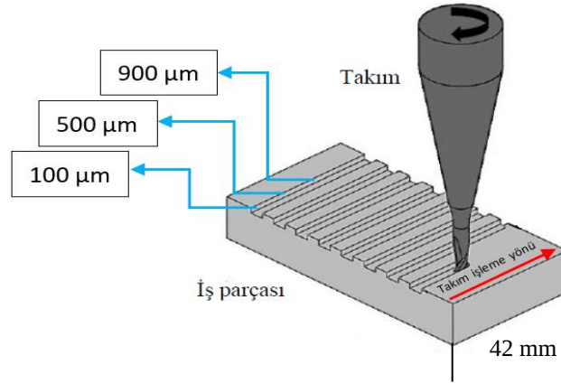
Resim 3. 5 Kesme mesafesi boyunca her kanalın belirli ölçü aralıklarında Ra ve Rz değerleri elde edilmesinin şematik gösterimi.
