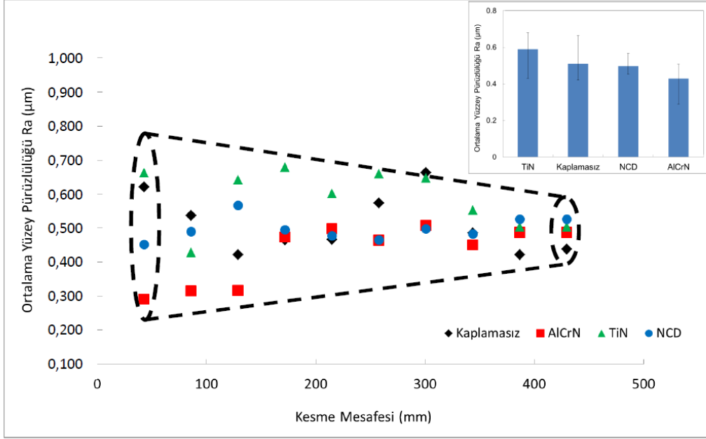
Şekil 2. 13 Kesme mesafesine ve kaplamalı-kaplamasız takımların türüne bağı olarak Ra değışimi (Hopa 2016).
