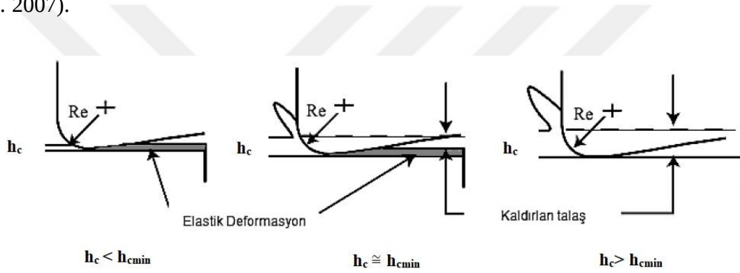
Şekil 2. 4 Minimum talaş kalınlığının etkilerinin şematik gösterimi (Chae et al. 2006).
