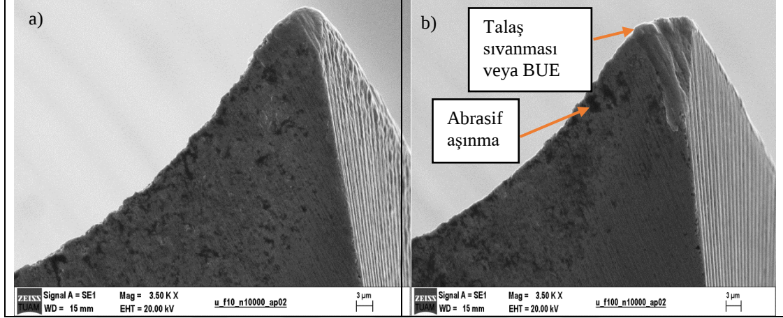
Şekil 4. 17 Kaplamasız takım için farklı ilerleme değerlerine bağlı olarak kenar radyüsünde meydana gelen aşınmaların görüntüleri (sabitler n=10\ 000 dev/dk., a_p=200\ \mu\text{m} ).
