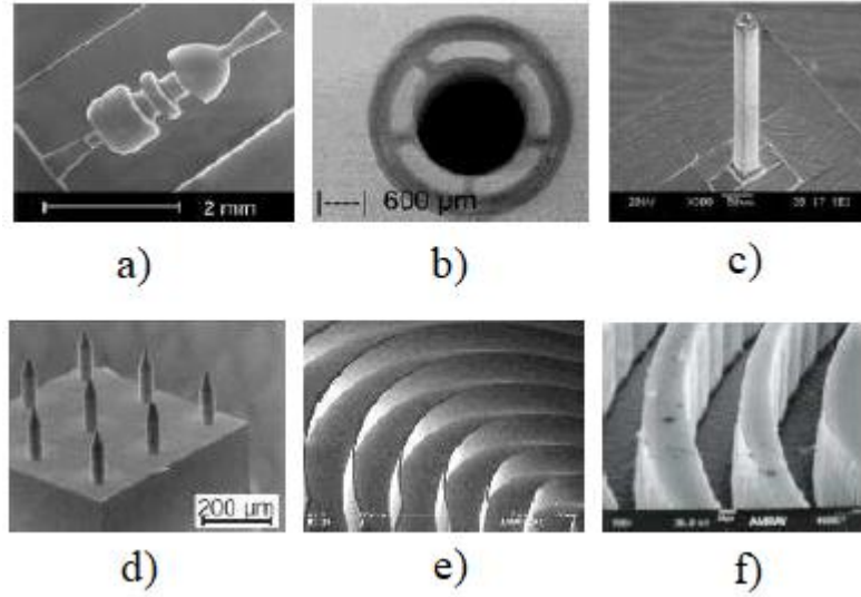
Şekil 1. 1 Mikro frezelem yöntemiyle üretilmiş bazı parça örnekleri a) ve b) Mikro Kalıplar (Çelik) (Brecher et al. 2008, Weule et al. 2001), c) ve d) Mikro Sütunlar (Pirinç) (Takeuchi et al. 2006, Bang et al. 2005), e) Mikro Duvarlar (Nikel Gümüş) (Weck et al. 2001), f) Mikro Siperler (PMMA, Friedrich et al. 1996).
