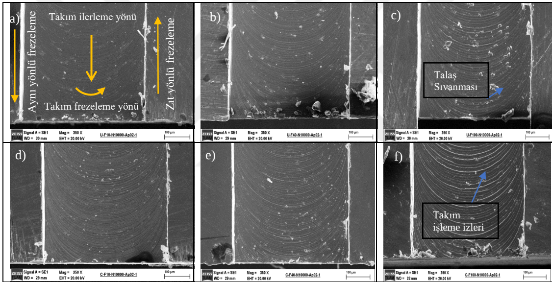
Şekil 4. 20 Kaplamasız ve elmas kaplanmış takımlar için farklı ilerleme değerlerinde elde edilen işlenmiş kanal görüntüleri (sabitler; n=10\ 000\ \text{dev/dk.} , a_p=200\ \mu\text{m} ).
