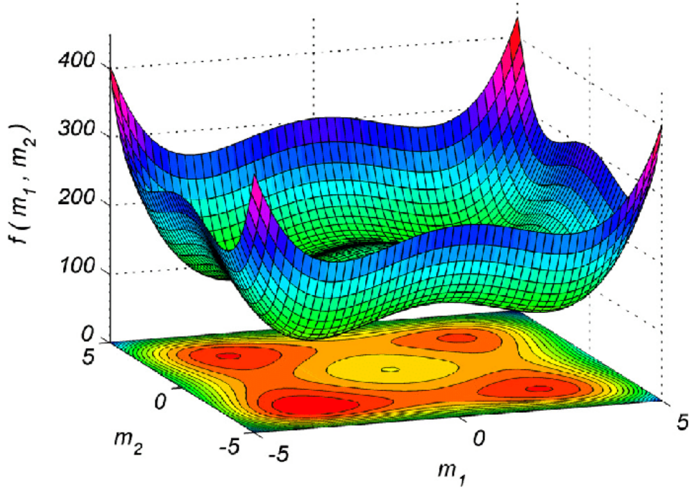
Şekil 3.8: Styblinski-Tang fonksiyonu 3-boyutlu görünümü.
