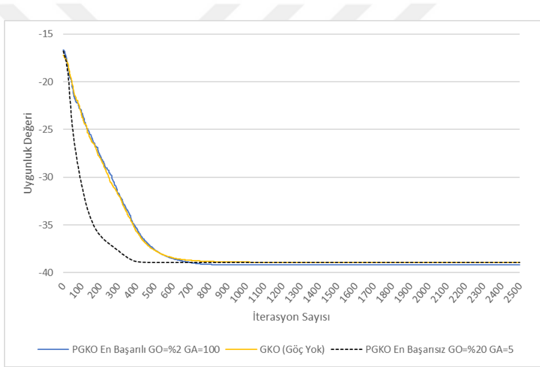
Şekil 4.11: Styblinski-Tang fonksiyonu global minimuma yakınsama grafiği.
