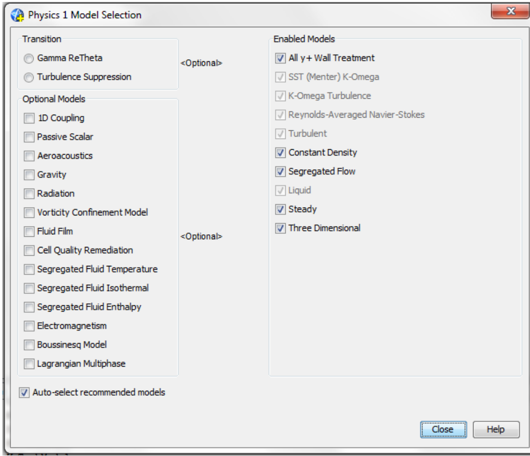
Şekil 5.16 : Fizik bölümünde seçilen matematiksel modeller.
