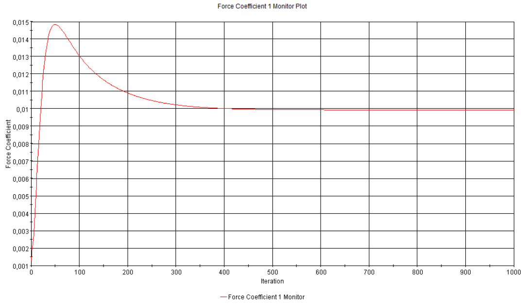
Şekil B. 13 : Pürüzlülük değeri k = 3000 \mu m olan plakanın sürtünme direnci katsayısı iterasyonları.
