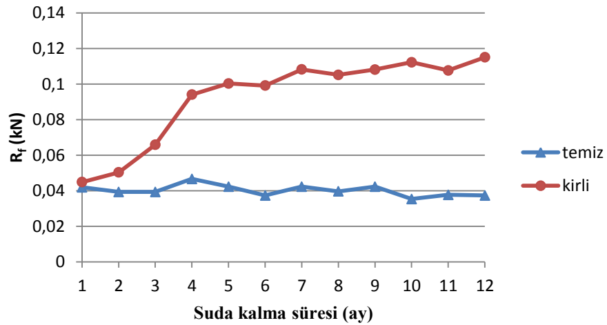
Şekil 4.19 : 2 knot hızında, fouling ’in sürtünme direnci üzerine etkisi (Taylan, 2010).
