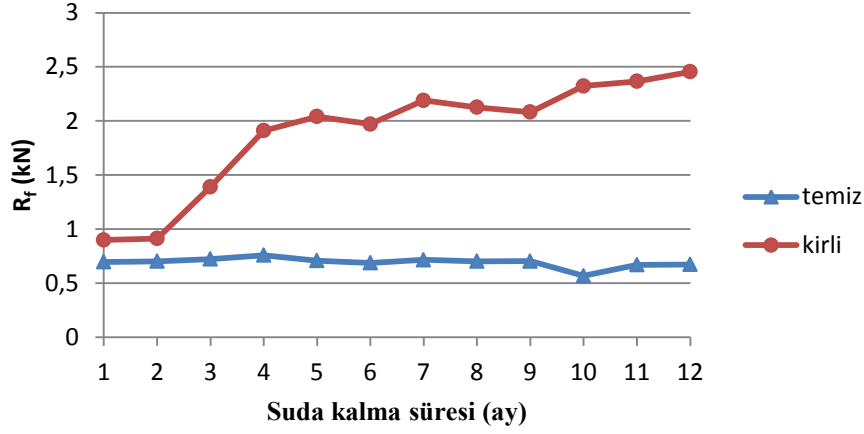
Şekil 4.20 : 9 knot hızında, fouling 'in sürtünme direnci üzerine etkisi (Taylan, 2010).
