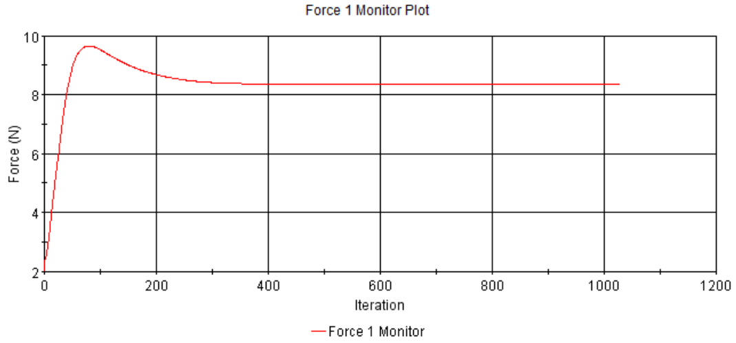
Şekil A. 8 : Pürüzlülük değeri k= 250 \mu m olan plakanın sürtünme direnci iterasyonları.
