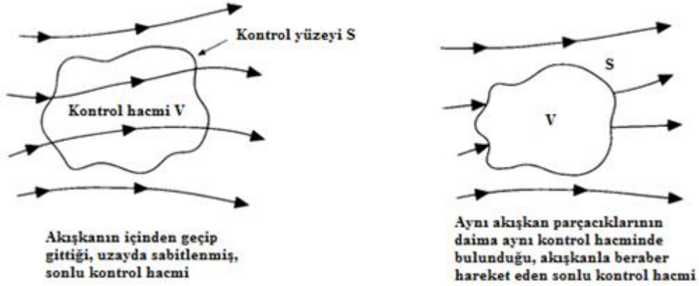
Şekil 3.10 : Sonlu kontrol hacmi için 2 farklı yaklaşım (Anderson J. D., 1995).
