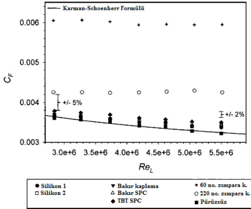
Şekil 4.27 : Temiz plakaların farklı Reynolds sayıları için bulunan sürtünme direnci katsayıları (Schultz, 2004).
