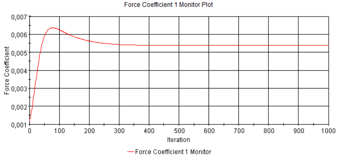
Şekil A. 13 : Pürüzlülük değeri k= 350 \mu m olan plakanın sürtünme direnci katsayısı iterasyonları.
