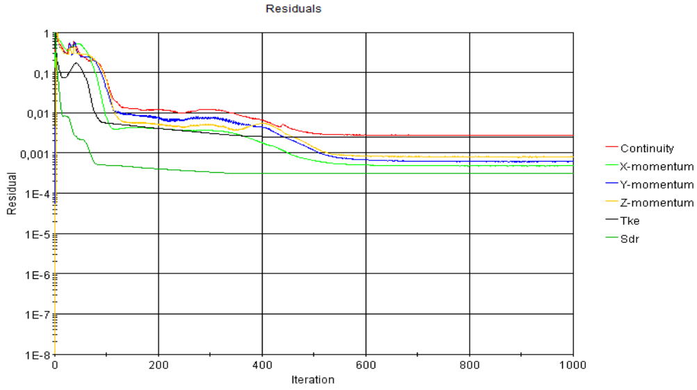
Şekil B. 12 : Pürüzlülük değeri k = 1000 \mu m olan plakanın analiz artık sonuçları iterasyonları.
