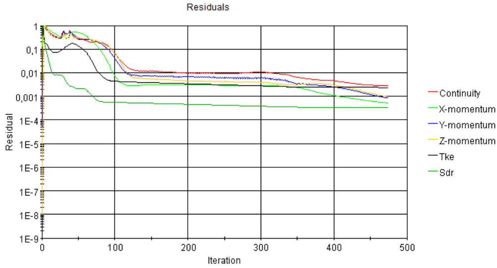
Şekil 5.23 : 60 numara zımpara kağıdı ile sarılmış plakanın analiz artık sonuçları iterasyonları.
