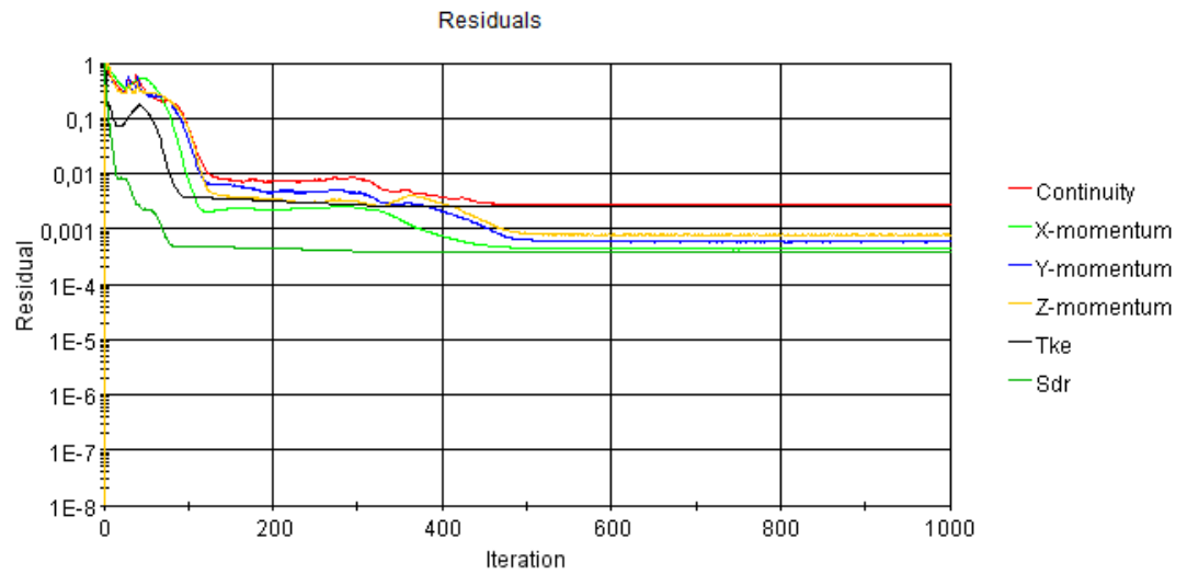
Şekil B. 6 : Pürüzlülük değeri k = 100 \mu m olan plakanın analiz artık sonuçları iterasyonları.
