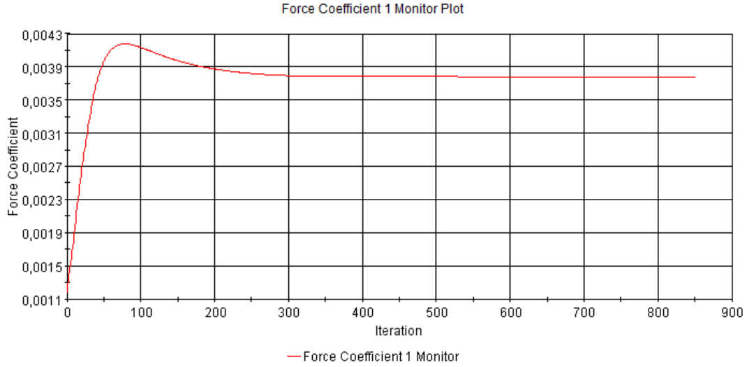
Şekil 5.27 : TBT SPC ile boyanmış plakanın sürtünme direnci katsayısı iterasyonları.
