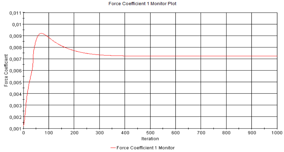
Şekil B. 10 : Pürüzlülük değeri k = 1000 \mu m olan plakanın sürtünme direnci katsayısı iterasyonları.
