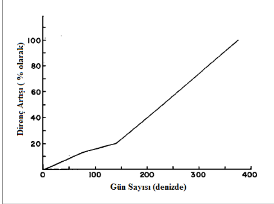
Şekil 4.22 : Yudachi direnç değerlerinin yüzde olarak artışı (Izubuchi, 1934).
