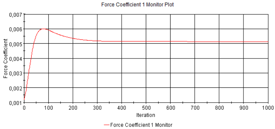
Şekil B. 7 : Pürüzlülük değeri k = 300 \mu m olan plakanın sürtünme direnci katsayısı iterasyonları.
