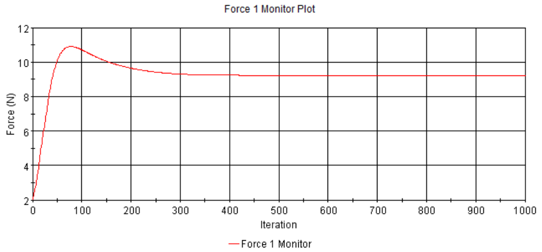
Şekil A. 14 : Pürüzlülük değeri k= 350 \mu m olan plakanın sürtünme direnci iterasyonları.
