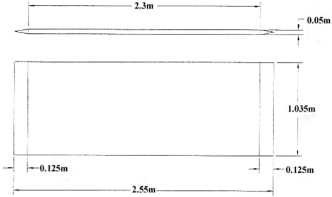
Şekil 4.23 : Deneyde kullanılan plakanın boyutları (Candries, 2001).
