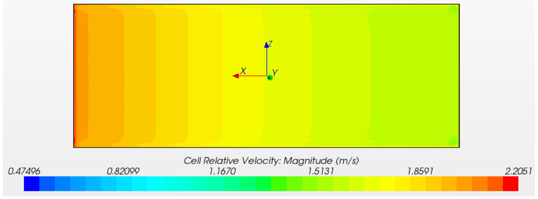
Şekil 5.43 : Global renk skalasına göre ağır kaygan çamur tabakası oluşumu durumunda yüzey yerel akış hızları.
