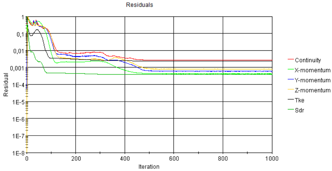
Şekil 5.20 : Pürüzsüz plaka analiz artık sonuçları iterasyonları.
