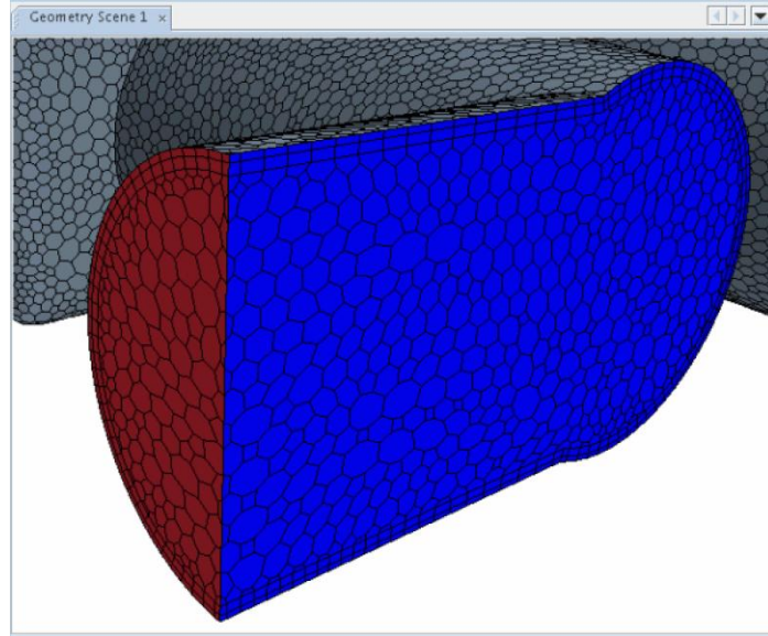
Şekil 5.15 : Prism layer mesher seçeneği ile oluşturulmuş sınır tabaka temsili (CD-ADAPCO, 2011).
