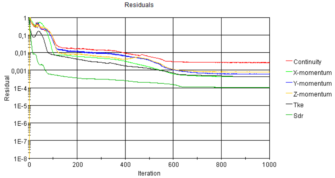
Şekil B. 18 : Pürüzlülük değeri k = 10000 \mu m olan plakanın analiz artık sonuçları iterasyonları.
