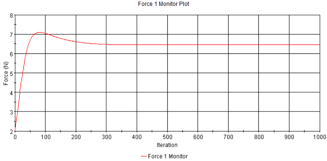
Şekil 5.19 : Pürüzsüz plakanın sürtünme direnci iterasyonları.
