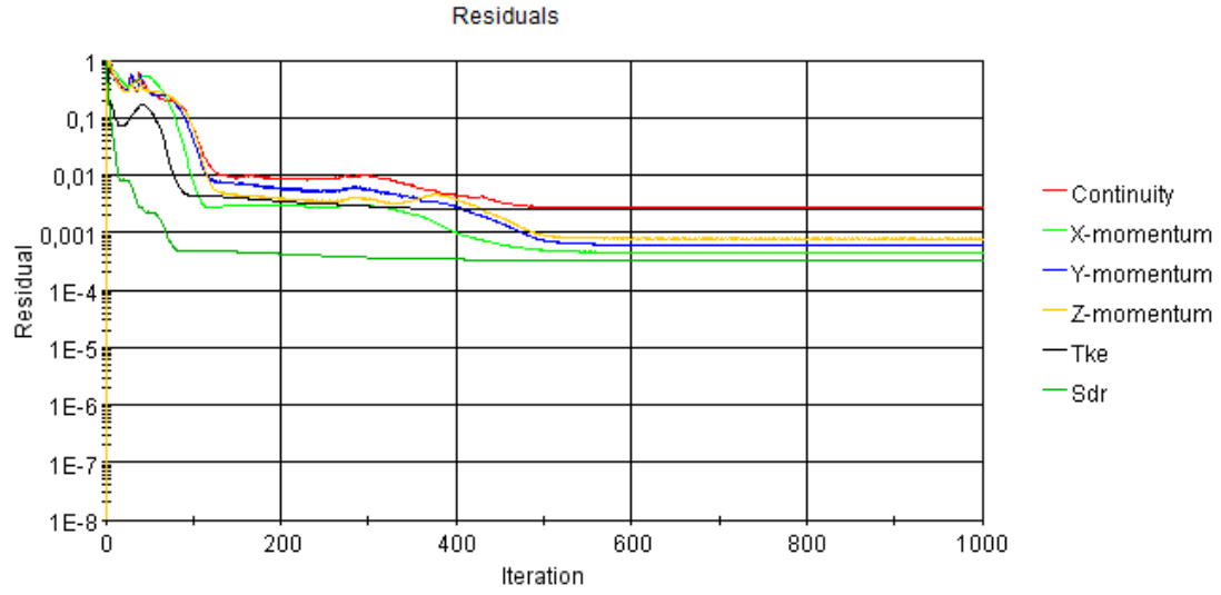
Şekil A. 12 : Pürüzlülük değeri k= 300 \mu m olan plakanın analiz artık sonuçları iterasyonları.
