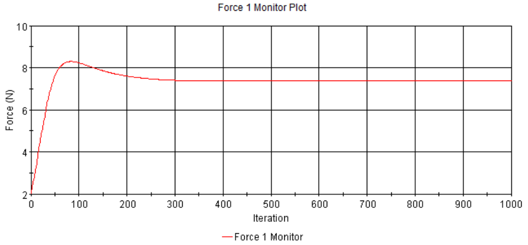
Şekil A. 5 : Pürüzlülük değeri k= 150 \mu m olan plakanın sürtünme direnci iterasyonları.
