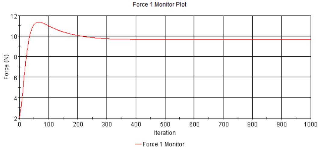
Şekil A. 29 : Pürüzlülük değeri k = 600 \mu m olan plakanın sürtünme direnci iterasyonları.
