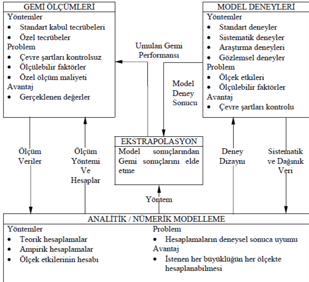
Şekil 3.4 : Gemi direnci incelemesinde bilgi akış çevirimi (Url-3).
