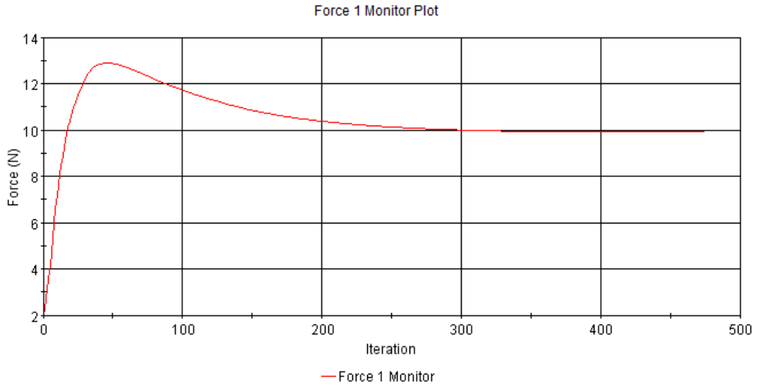
Şekil 5.22 : 60 numara zımpara kağıdı ile sarılmış plakanın sürtünme direnci iterasyonları.
