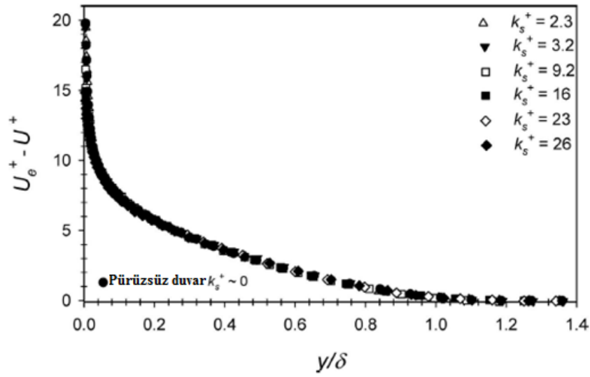
Şekil 4.17 : Farklı pürüzlülük Reynolds sayılarının dış katmandaki etkileri (Schultz ve Flack, 2007).
