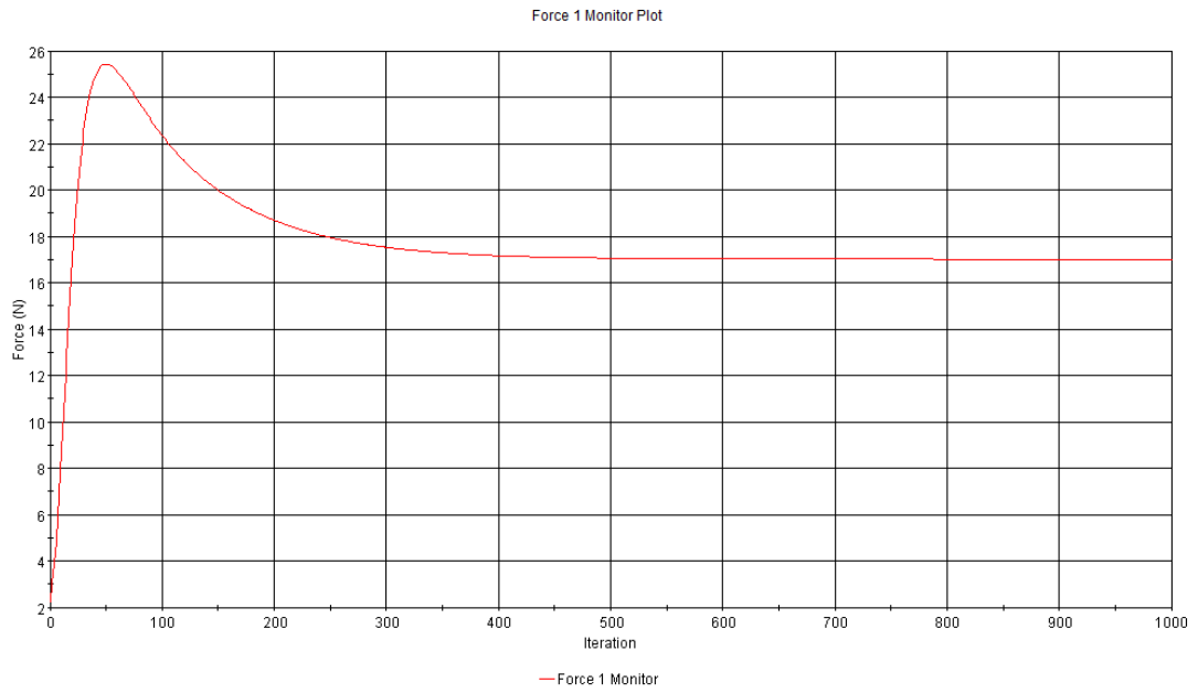
Şekil B. 14 : Pürüzlülük değeri k = 3000 \mu m olan plakanın sürtünme direnci iterasyonları.
