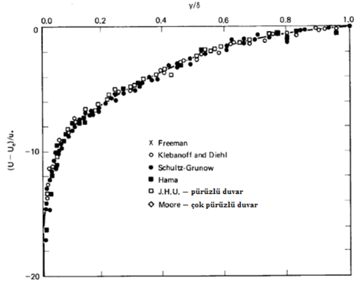
Şekil 4.12 : Pürüzlü ve pürüzsüz düz plakalar için türbülans sınır tabaka dış bölgede hız sapma kanunu (Schetz, 1993).
