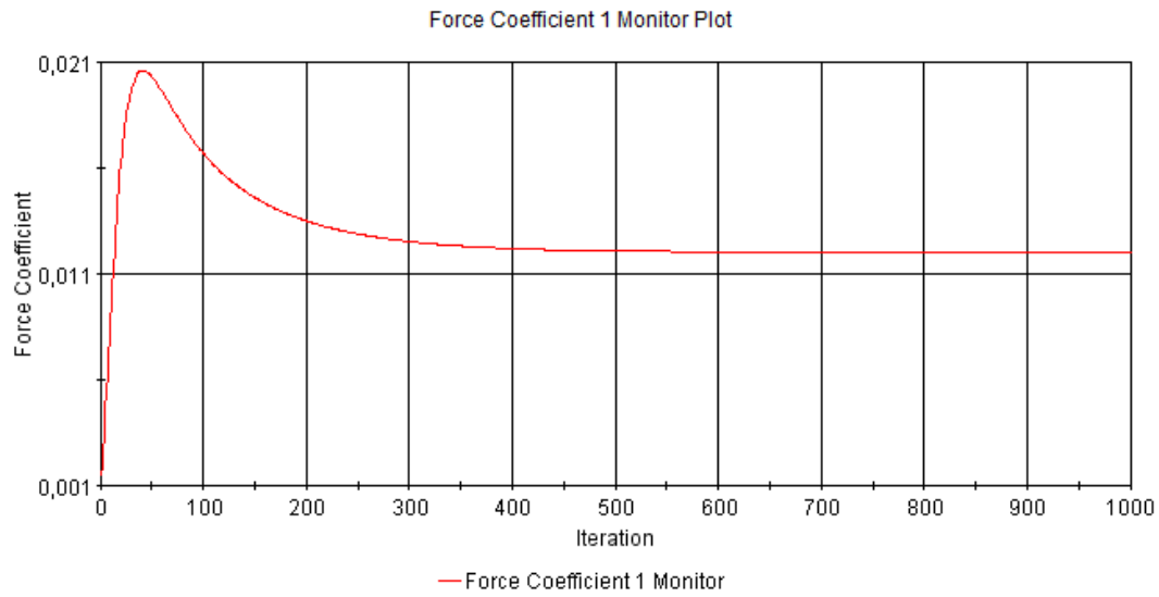
Şekil B. 16 : Pürüzlülük değeri k = 10000 \mu m olan plakanın sürtünme direnci katsayısı iterasyonları.
