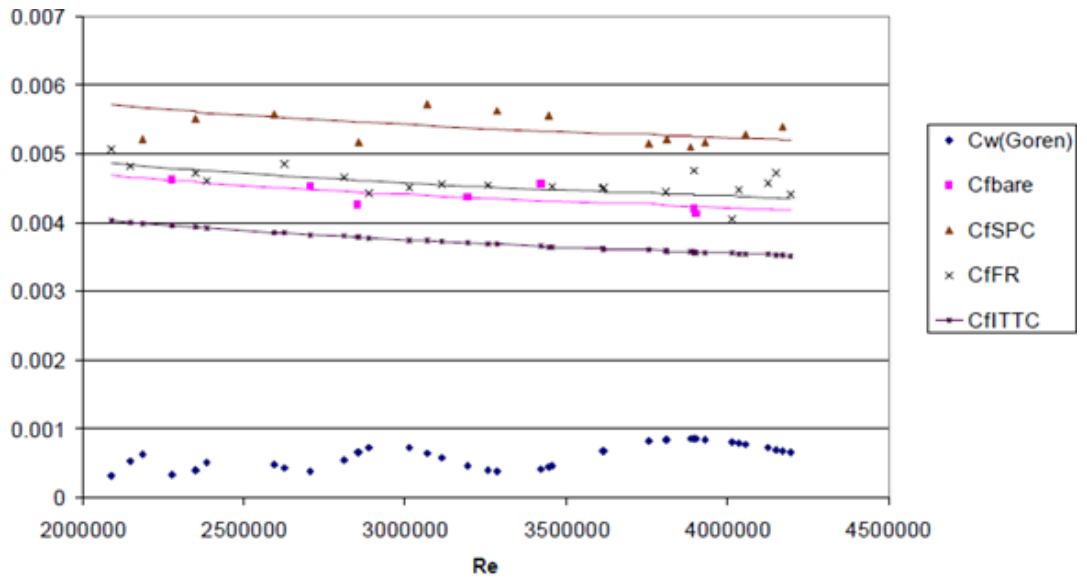
Şekil 4.25 : Farklı Reynolds sayıları için bulunan sürtünme direnci ve dalga direnci katsayıları (Candries, 2001).
