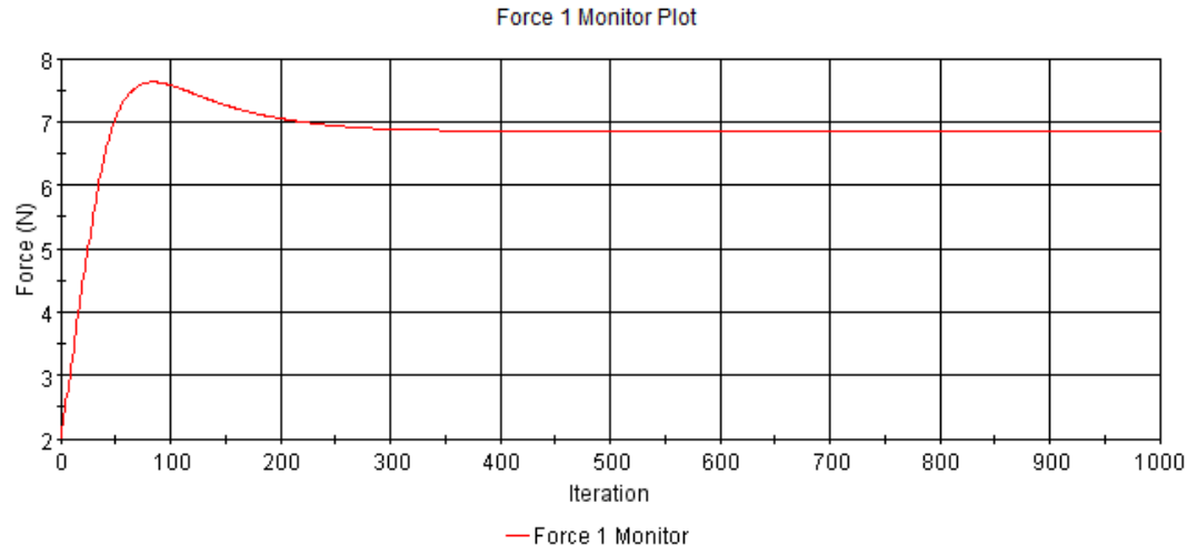
Şekil A. 2 : Pürüzlülük değeri k=100 \mu m olan plakanın sürtünme direnci iterasyonları.
