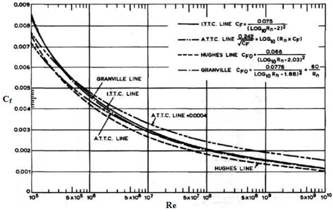
Şekil 3.3 : Yüzey sürtünmesi eğrileri (Lewis E. , 1988).
