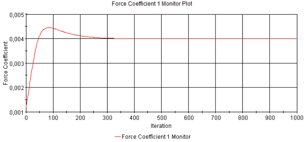
Şekil A. 1 : Pürüzlülük değeri k=100 \mu m olan plakanın sürtünme direnci katsayısı iterasyonları.
