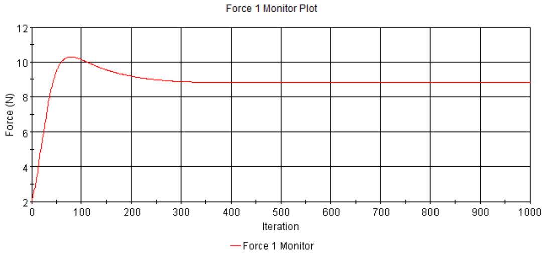
Şekil B. 8 : Pürüzlülük değeri k = 300 \mu m olan plakanın sürtünme direnci iterasyonları.
