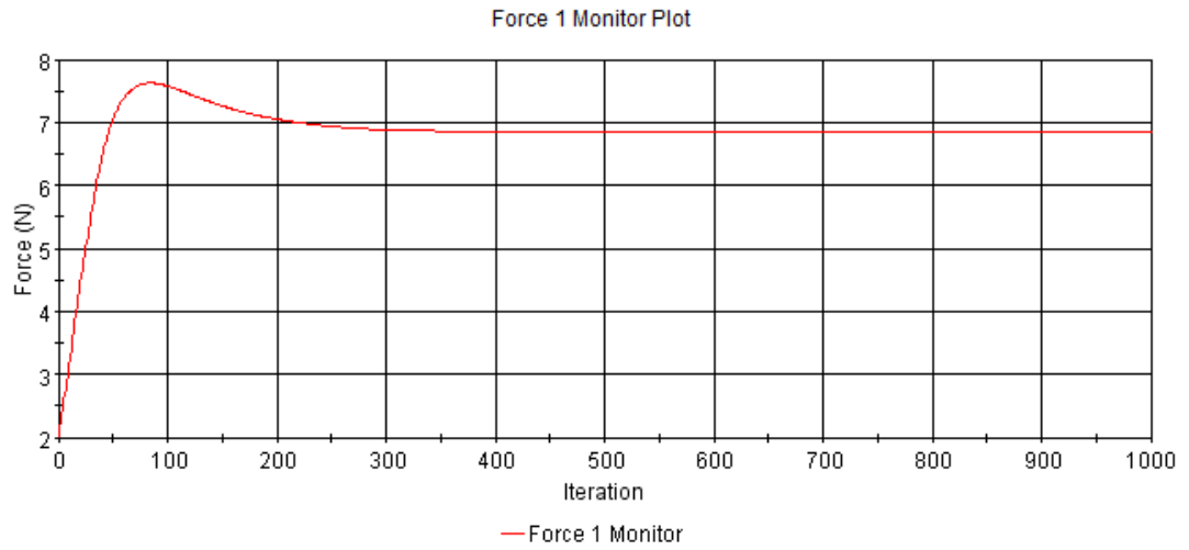
Şekil B. 5 : Pürüzlülük değeri k = 100 \mu m olan plakanın sürtünme direnci iterasyonları.
