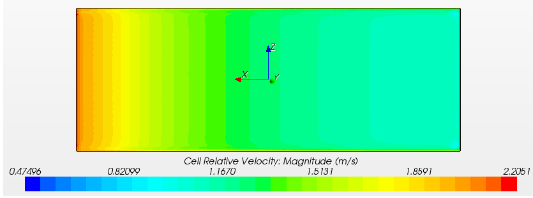
Şekil 5.46 : Global renk skalasına göre ağır kalkerli fouling durumunda yüzey yerel akış hızları.
