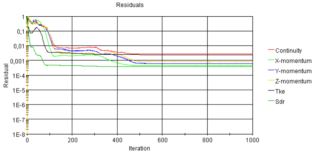
Şekil B. 3 : Pürüzlülük değeri k = 30 \mu m olan plakanın analiz artık sonuçları iterasyonları.
