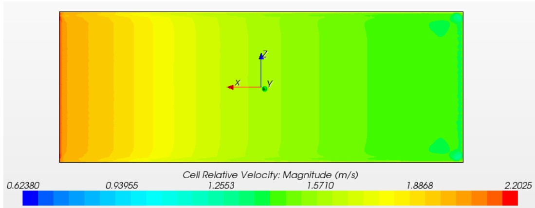
Şekil 5.37 : Hafif kalkerli veya yosunlu fouling durumunda yüzey yerel akış hızları.
