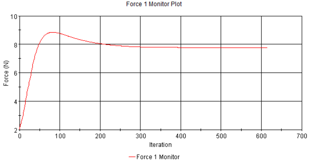
Şekil 5.25: 220 numara zımpara kağıdı ile sarılmış plakanın sürtünme direnci iterasyonları.
