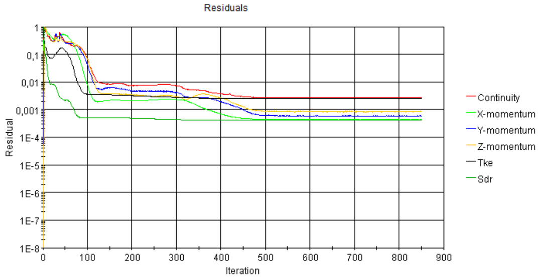
Şekil 5.29 : TBT SPC ile boyanmış plakanın analiz artık sonuçları iterasyonları.
