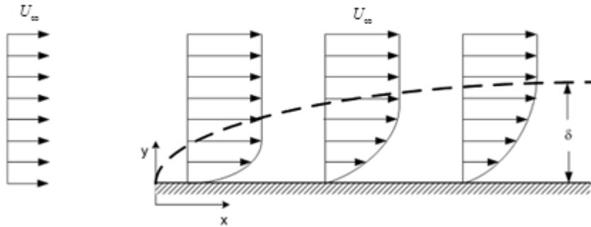
Şekil 4.6: Sınır tabaka kalınlığı \delta ve hız profilinin değişimi (Url-6).
