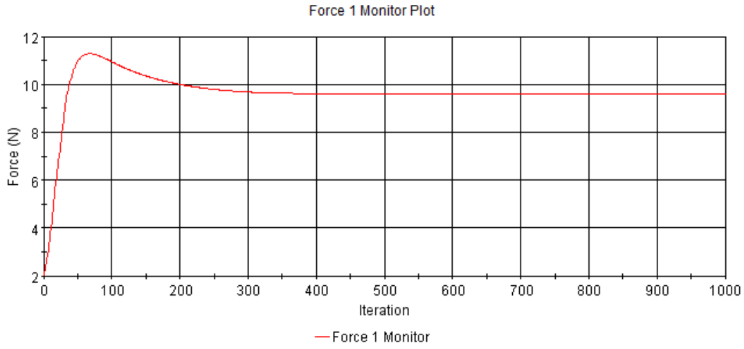
Şekil A. 23 : Pürüzlülük değeri k= 500 \mu m olan plakanın sürtünme direnci iterasyonları.
