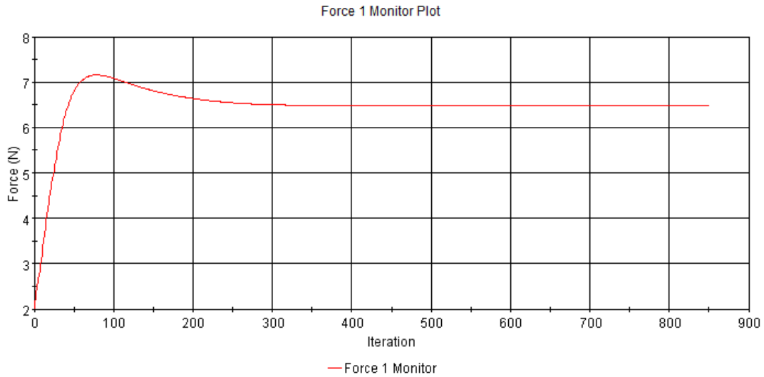
Şekil 5.28 : TBT SPC ile boyanmış plakanın sürtünme direnci iterasyonları.
