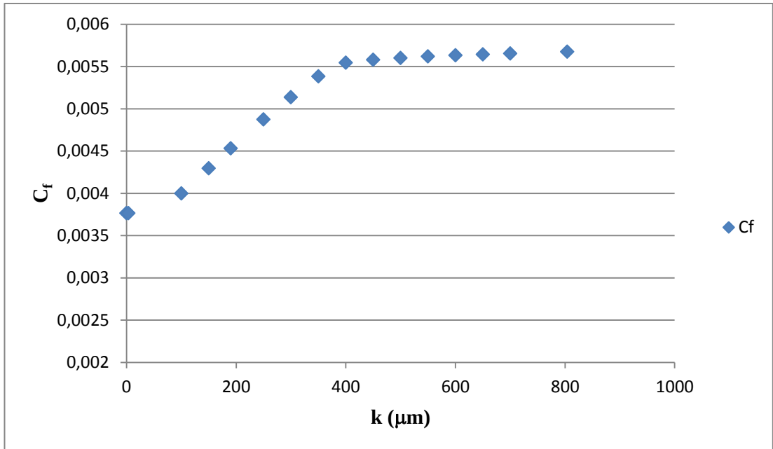
Şekil 5.31 : Parametrik analiz sonucu bulunan farklı pürüzlülük değerlerine karşılık gelen sürtünme direnci katsayıları.
