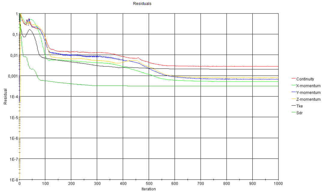
Şekil B. 15 : Pürüzlülük değeri k = 3000 \mu m olan plakanın analiz artık sonuçları iterasyonları.
