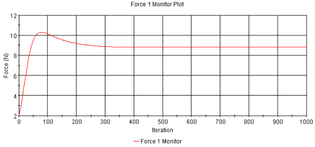
Şekil A. 11 : Pürüzlülük değeri k= 300 \mu m olan plakanın sürtünme direnci iterasyonları.
