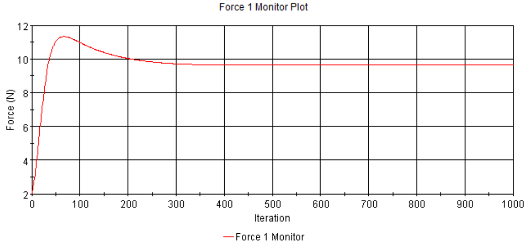
Şekil A. 26 : Pürüzlülük değeri k= 550 \mu m olan plakanın sürtünme direnci iterasyonları.
