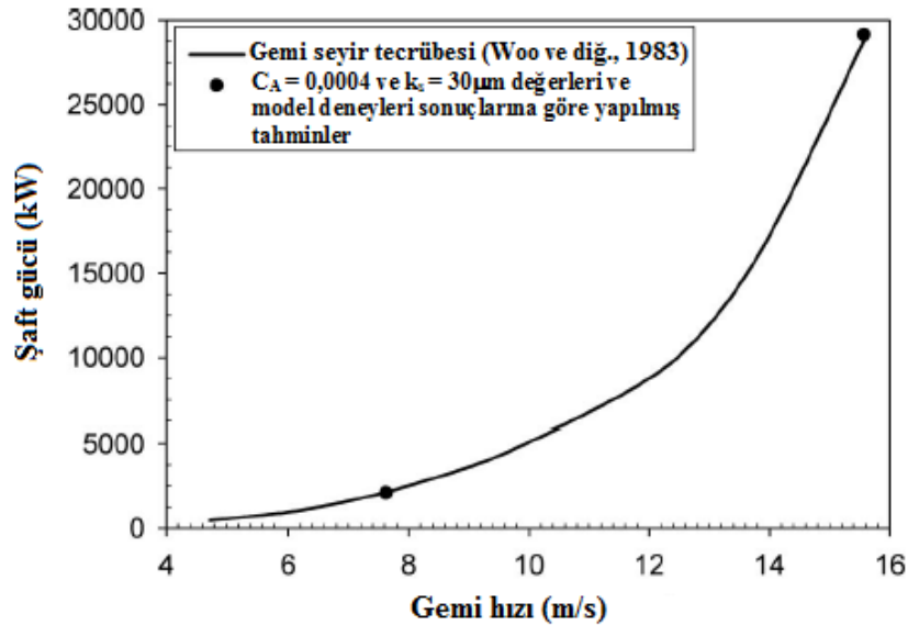
Şekil 4.32 : k_s = 30 \mu m için farklı hızlardaki gerekli şaft gücü miktarları (Schultz, 2007).
