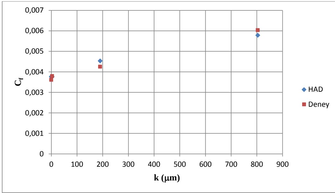
Şekil 5.30 : Doğrulama için HAD ile bulunan sürtünme direnci katsayısı değerleriyle deneylerde bulunan sürtünme direnci katsayısı değerlerinin karşılaştırılması.
