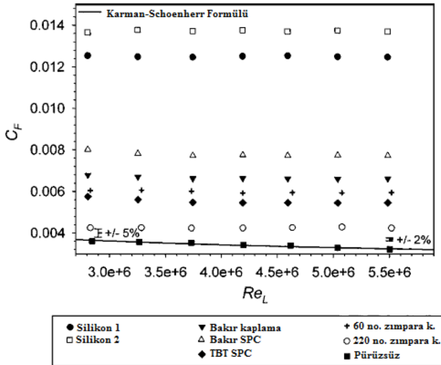
Şekil 4.28 : 287 gün boyunca fouling 'e maruz kalmış plakaların farklı Reynolds sayıları için bulunan sürtünme direnci katsayıları (Schultz, 2004).
