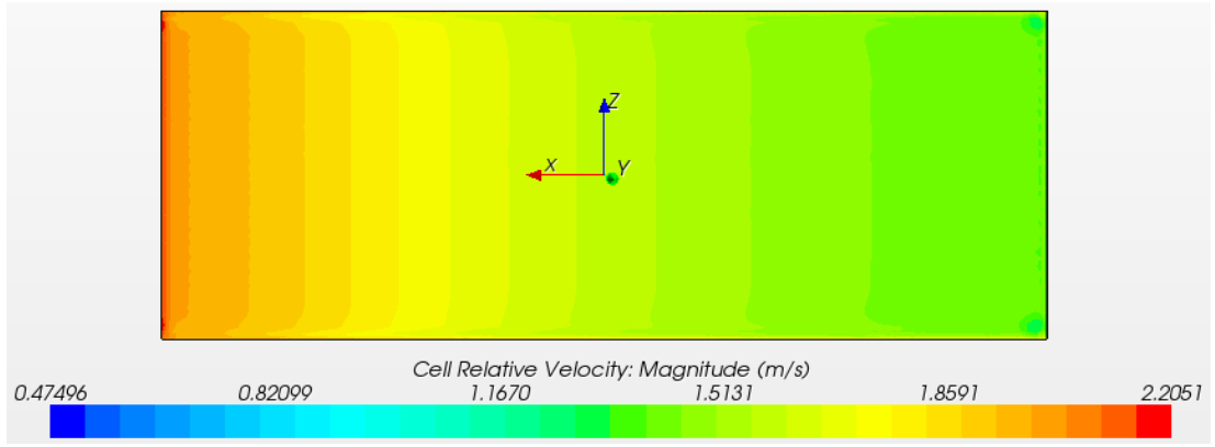
Şekil 5.44 : Global renk skalasına göre hafif kalkerli veya yosunlu fouling durumunda yüzey yerel akış hızları.
