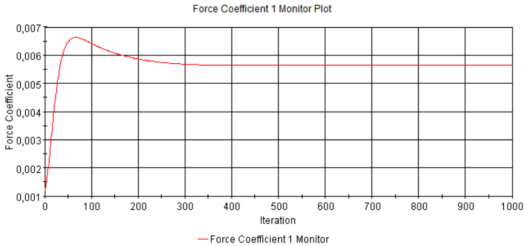
Şekil A. 28 : Pürüzlülük değeri k= 600 \mu m olan plakanın sürtünme direnci katsayısı iterasyonları.
