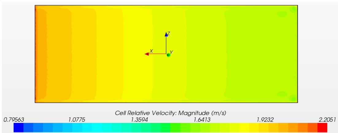
Şekil 5.34 : Antifouling boya uygulanmış yüzey yerel akış hızları.
