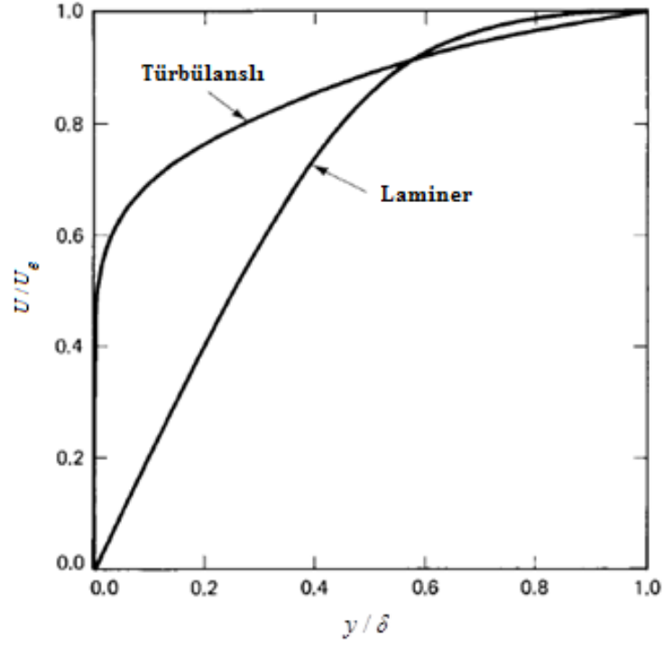
Şekil 4.8 : Laminar ve türbülans sınır tabaka hız profilleri (Schetz, 1993).
