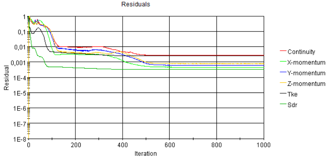
Şekil A. 21 : Pürüzlülük değeri k= 450 \mu m olan plakanın analiz artık sonuçları iterasyonları.
