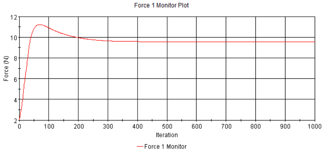
Şekil A. 20 : Pürüzlülük değeri k= 450 \mu m olan plakanın sürtünme direnci iterasyonları.
