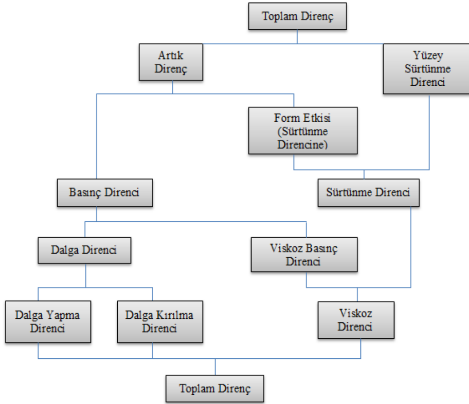
Şekil 3.1 : Gemi direnci bileşenleri (Carlton, 2007).
