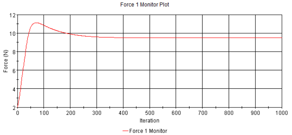
Şekil A. 17 : Pürüzlülük değeri k= 400 \mu m olan plakanın sürtünme direnci iterasyonları.
