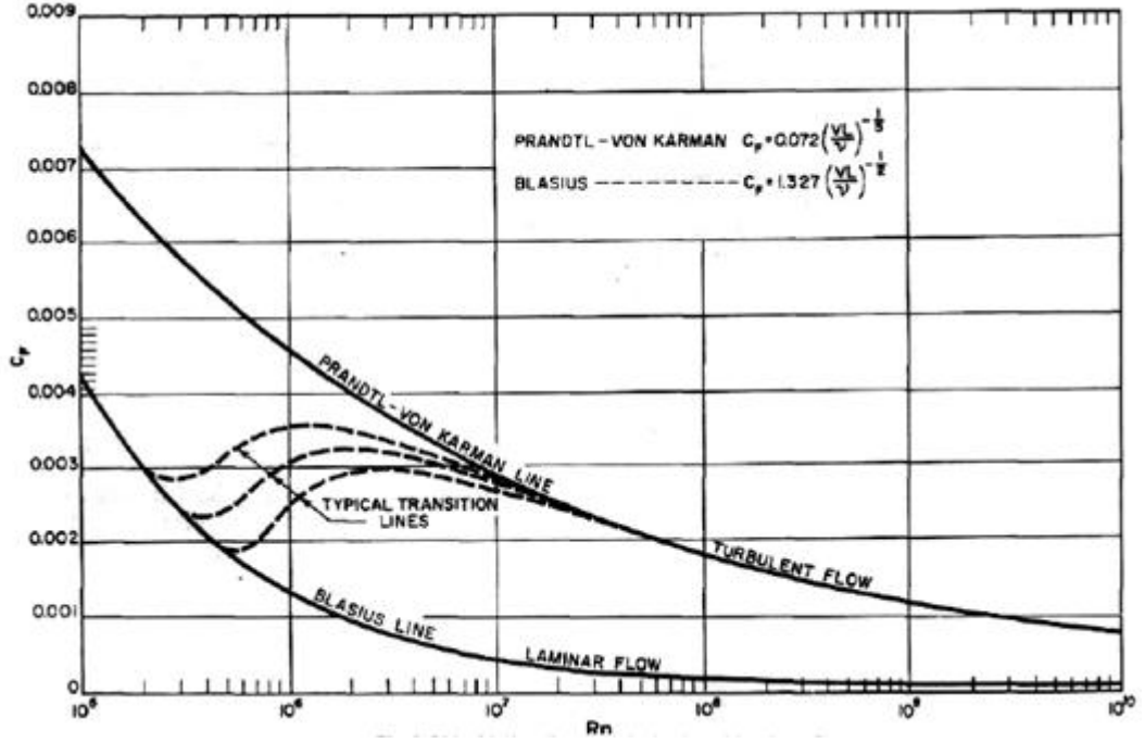
Şekil 3.2 : Türlölanslı ve laminar akışlar için yüzey sürtünme eğrileri. (Lewis E. , 1988).
