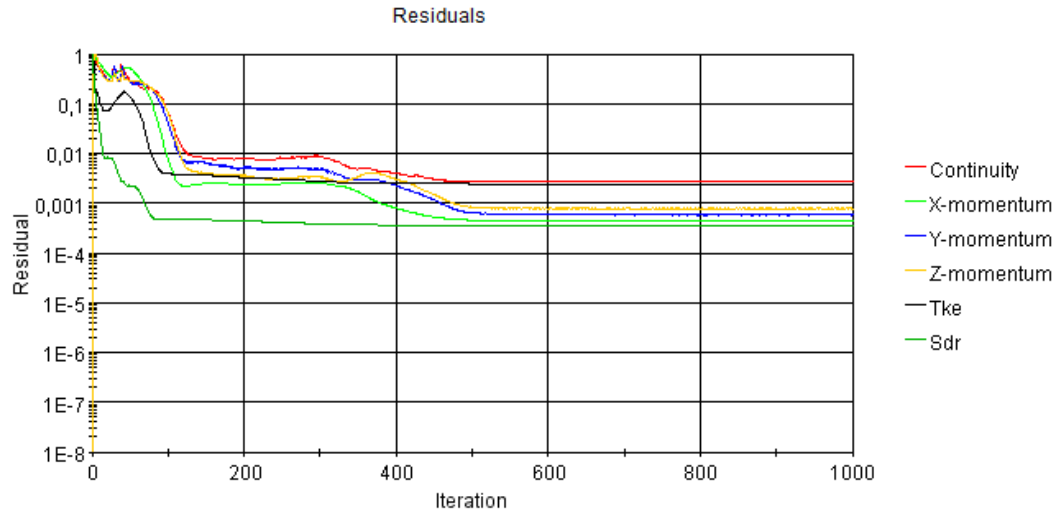
Şekil A. 6 : Pürüzlülük değeri k= 150 \mu m olan plakanın analiz artık sonuçları iterasyonları.
