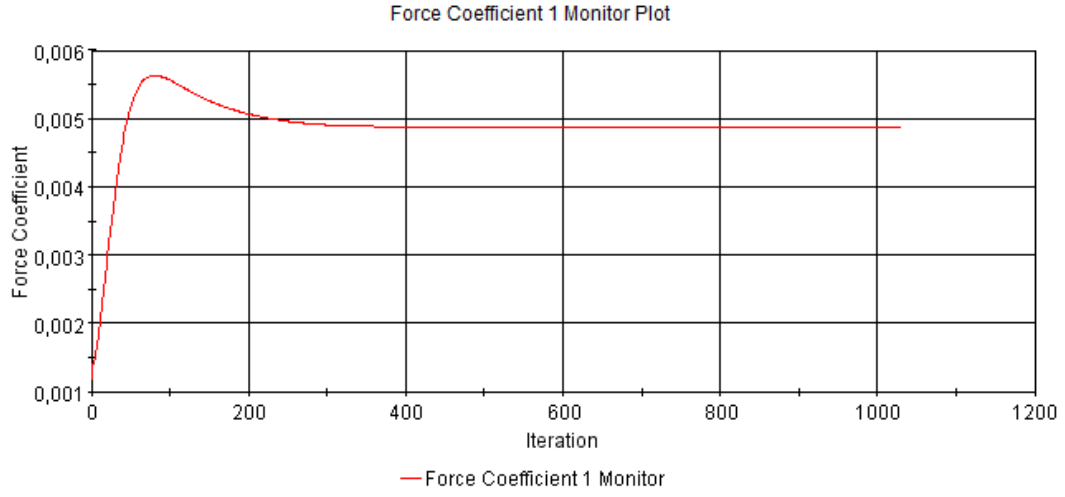
Şekil A. 7 : Pürüzlülük değeri k= 250 \mu m olan plakanın sürtünme direnci katsayısı iterasyonları.
