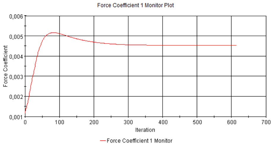
Şekil 5.24 : 220 numara zımpara kağıdı ile sarılmış plakanın sürtünme direnci katsayısı iterasyonları.
