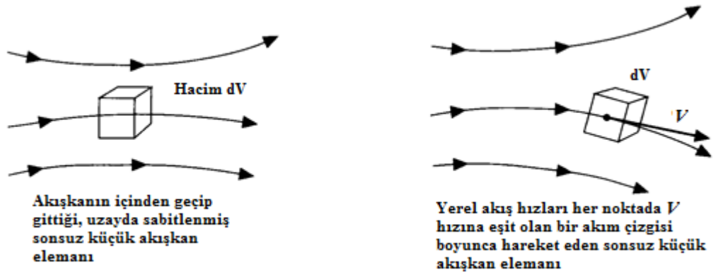
Şekil 3.11 : Sonsuz küçük akışkan elemanı için 2 farklı yaklaşım (Anderson J. D., 1995).
