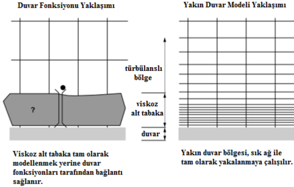
Şekil 5.17 : Yakın duvar modeli ve duvar fonksiyonu yaklaşımı (ANSYS, 2011).
