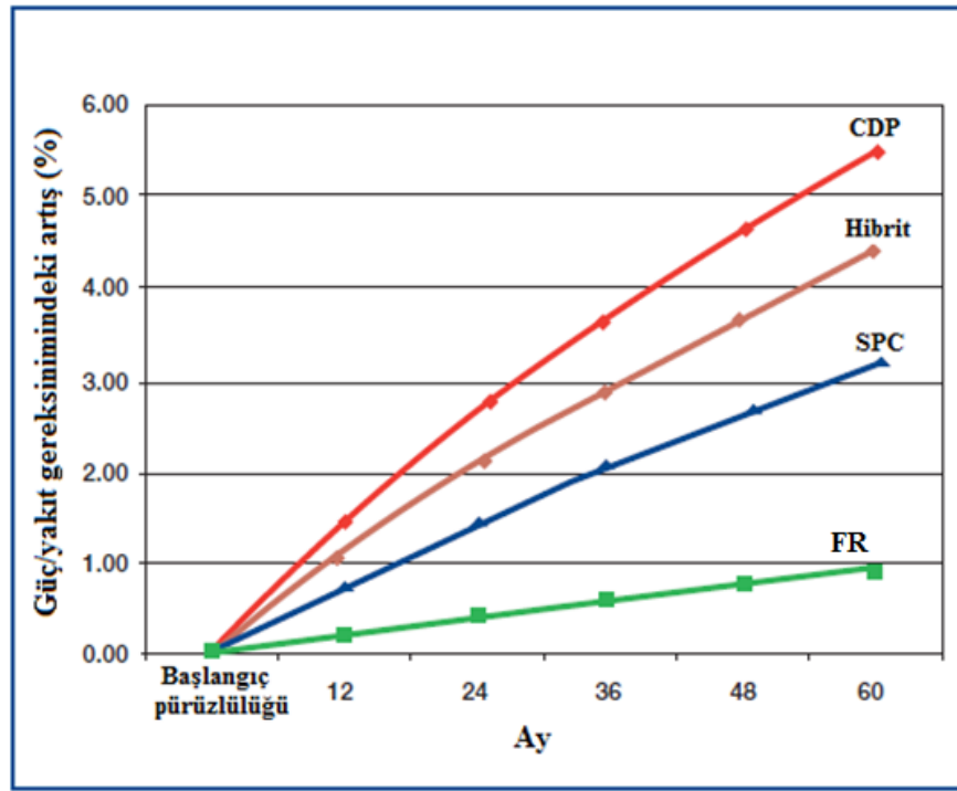
Şekil 2.5 : Farklı antifouling boyalarının zaman içerisinde artan pürüzlülük değerleri nedeniyle hızlı bir geminin zamana bağlı güç veya yakıt gereksinimindeki artış tahmini (Url-2).
