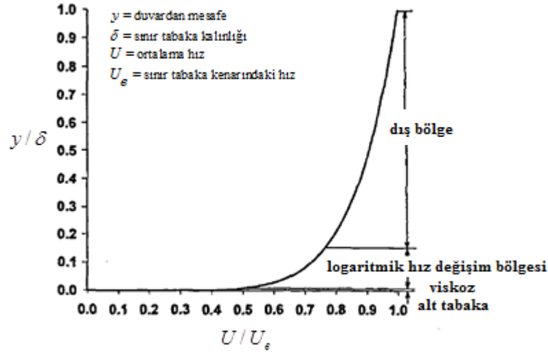
Şekil 4.11 : Türbülans sınır tabaka hız profili (Schultz, 2007).
