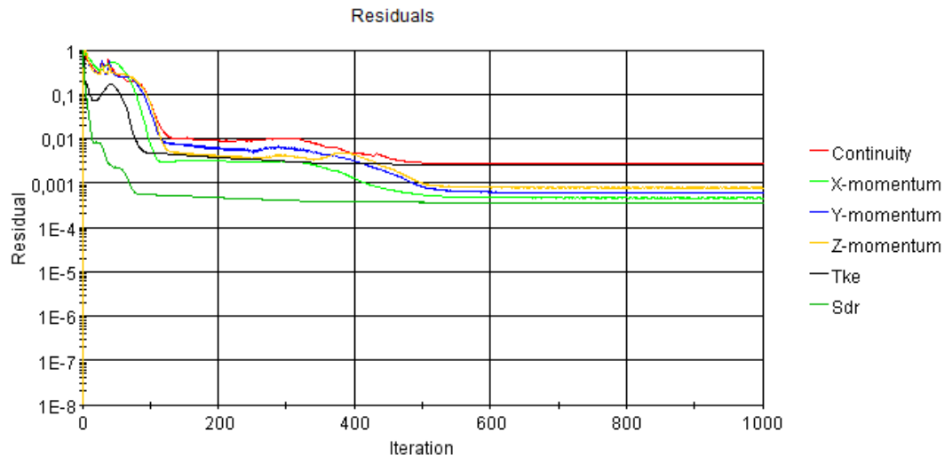
Şekil A. 30 : Pürüzlülük değeri k = 600 \mu m olan plakanın analiz artık sonuçları iterasyonları.
