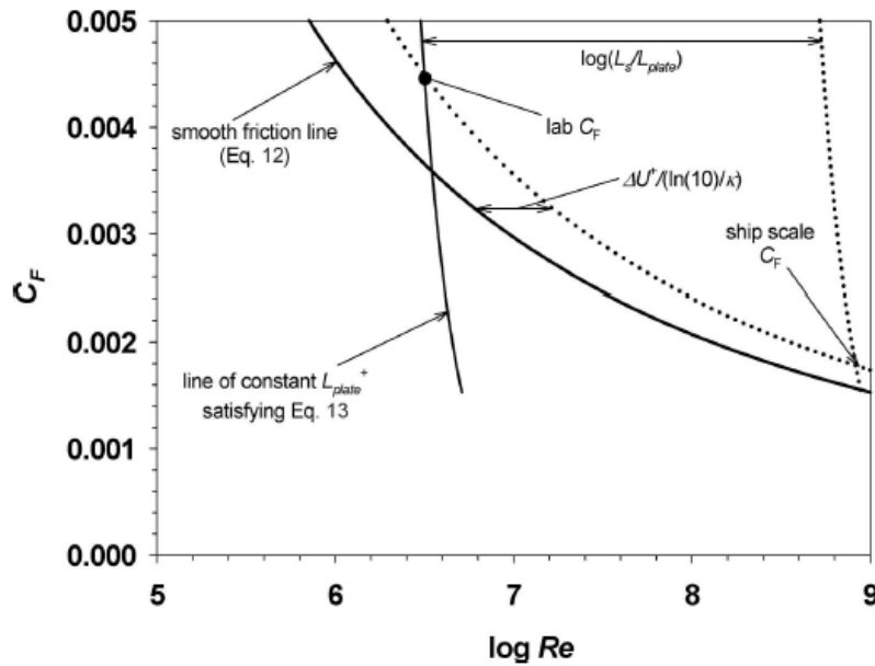
Şekil 4.31: Granville benzerlik kanunu prosedürü (Schultz, 2007).
