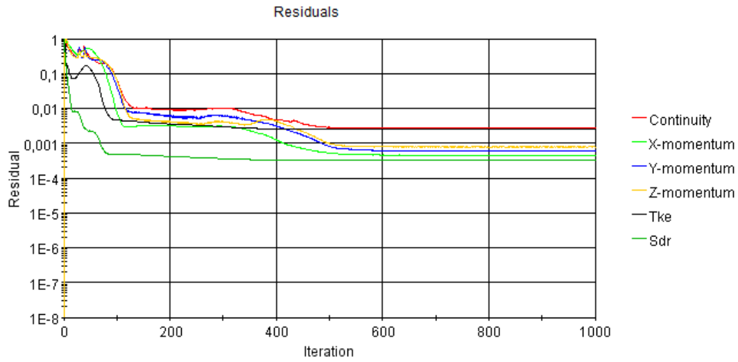
Şekil A. 24 : Pürüzlülük değeri k= 500 \mu m olan plakanın analiz artık sonuçları iterasyonları.
