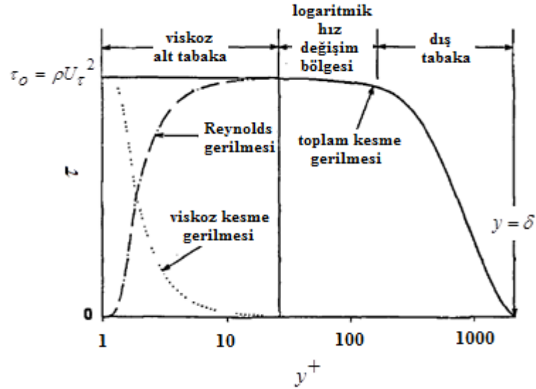
Şekil 4.13 : Türbülans sınır tabaka kesme gerilmeleri profili.
