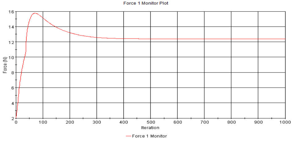
Şekil B. 11 : Pürüzlülük değeri k = 1000 \mu m olan plakanın sürtünme direnci iterasyonları.
