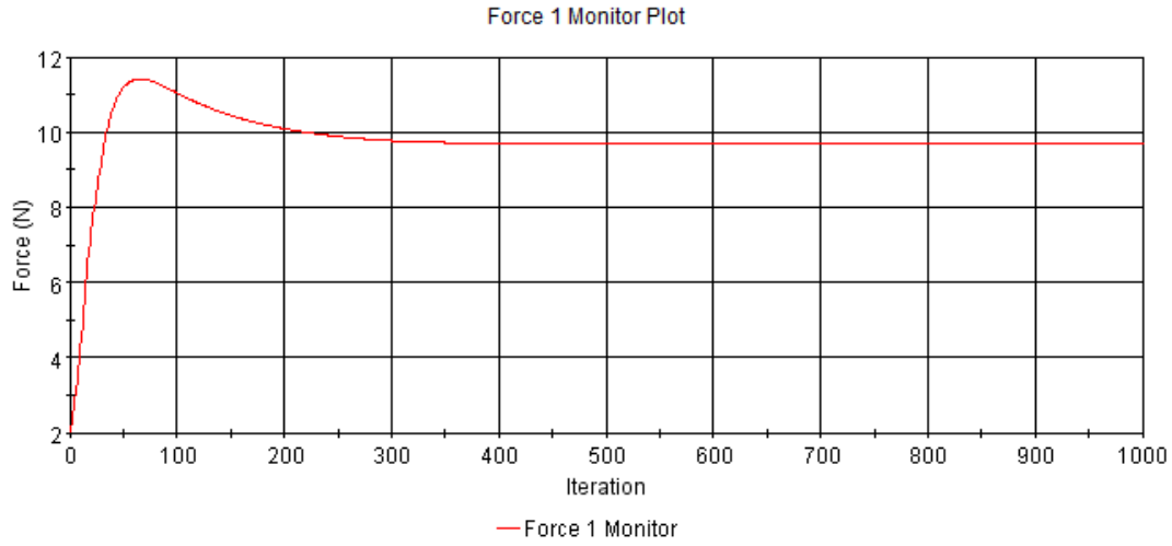
Şekil A. 35 : Pürüzlülük değeri k = 700 \mu m olan plakanın sürtünme direnci iterasyonları.
