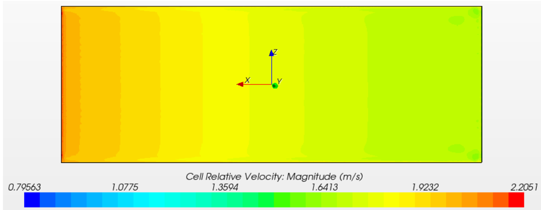
Şekil 5.33 : Pürüzsüz yüzey yerel akış hızları.
