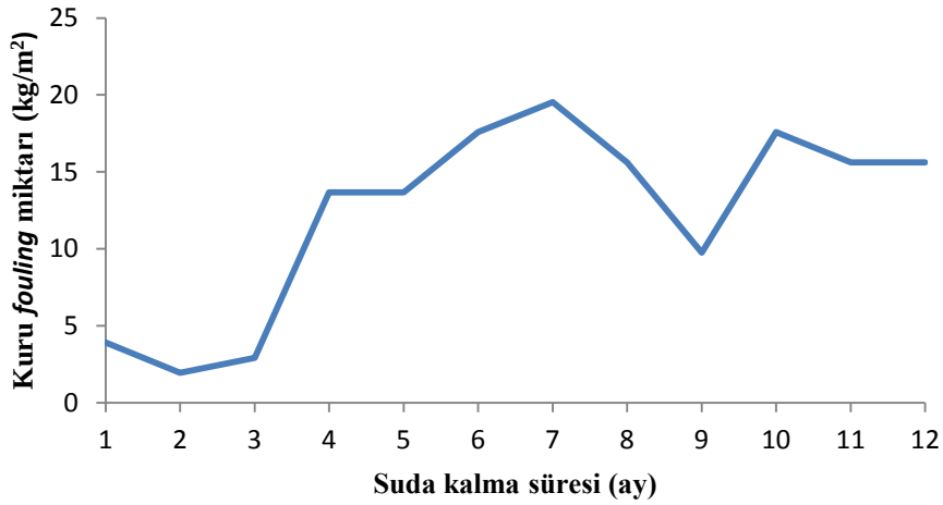
Şekil 4.18 : Test plakaları üzerindeki kuru fouling miktarı (Taylan, 2010).
