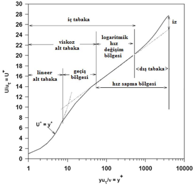
Şekil 4.10 : Türbülans sınır tabakada duvar kanunu (Schultz, 2007).
