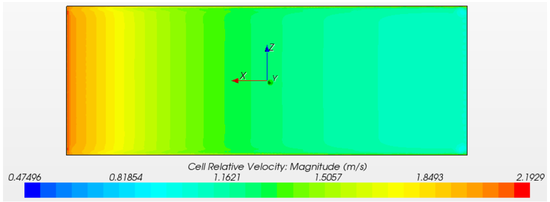
Şekil 5.39 : Ağır kalkerli fouling durumunda yüzey yerel akış hızları.
