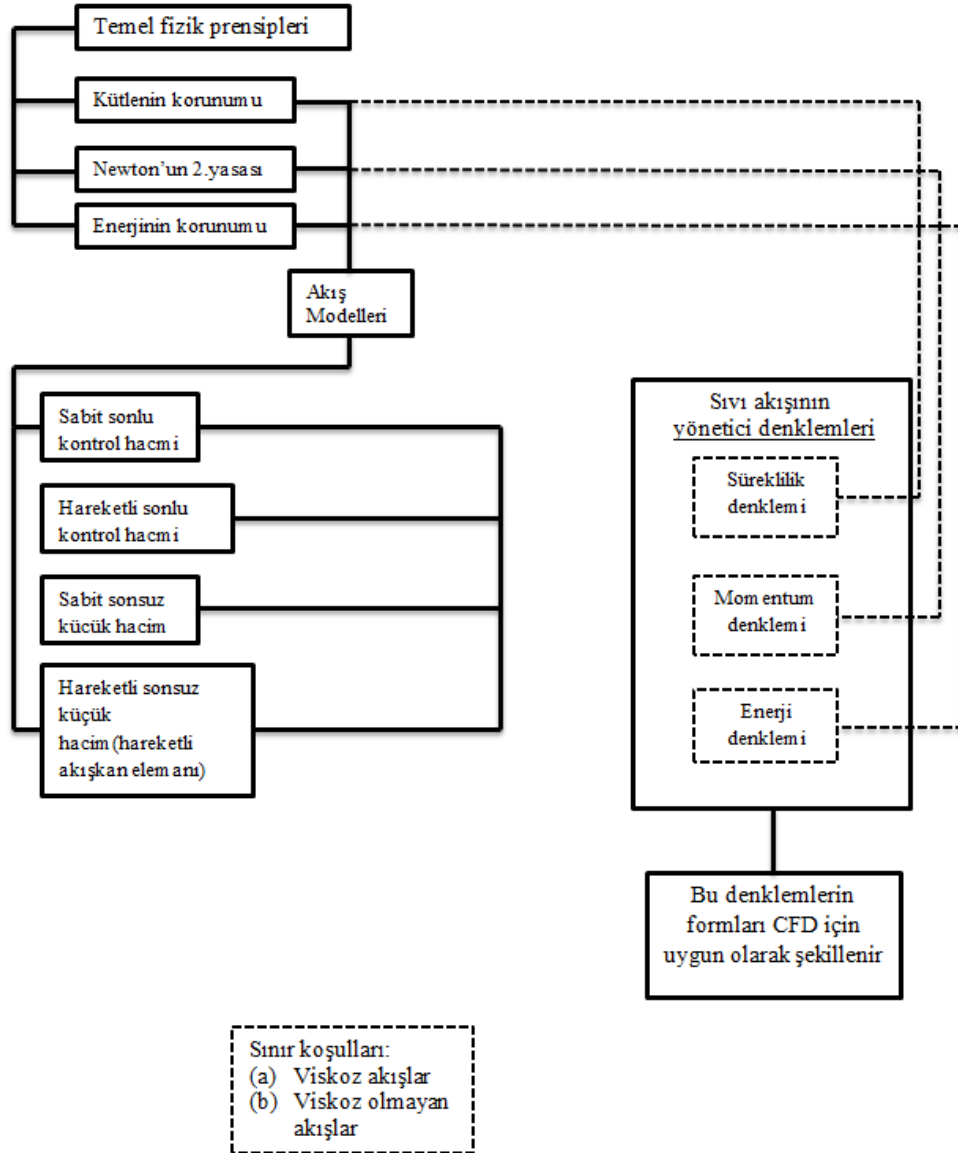
Şekil 3.9 : Hesaplamalı akışkanlar dinamiği algoritması (Anderson J. D., 1995).
