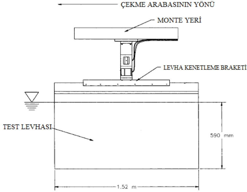
Şekil 4.26 : Deney düzeneği ve plaka (Schultz, 2004).
