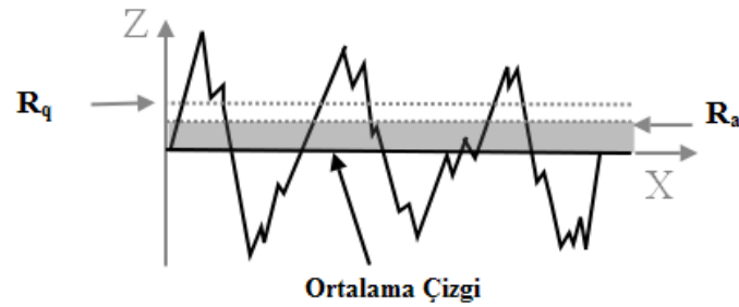
Şekil 4.5 : Ortalama pürüzlülük ve ortalama karekök pürüzlülüğünün temsili gösterimi (Url-5).
