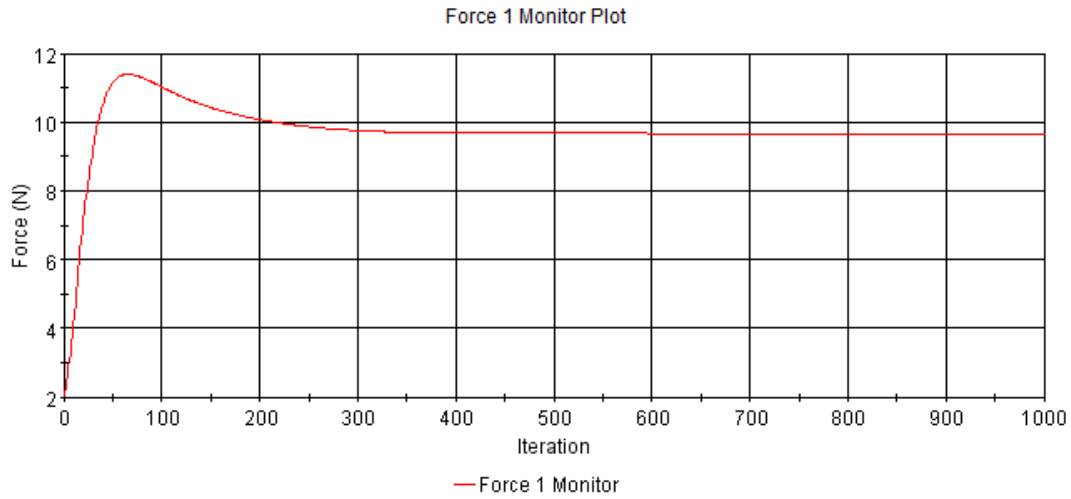
Şekil A. 32 : Pürüzlülük değeri k = 650 \mu m olan plakanın sürtünme direnci iterasyonları.
