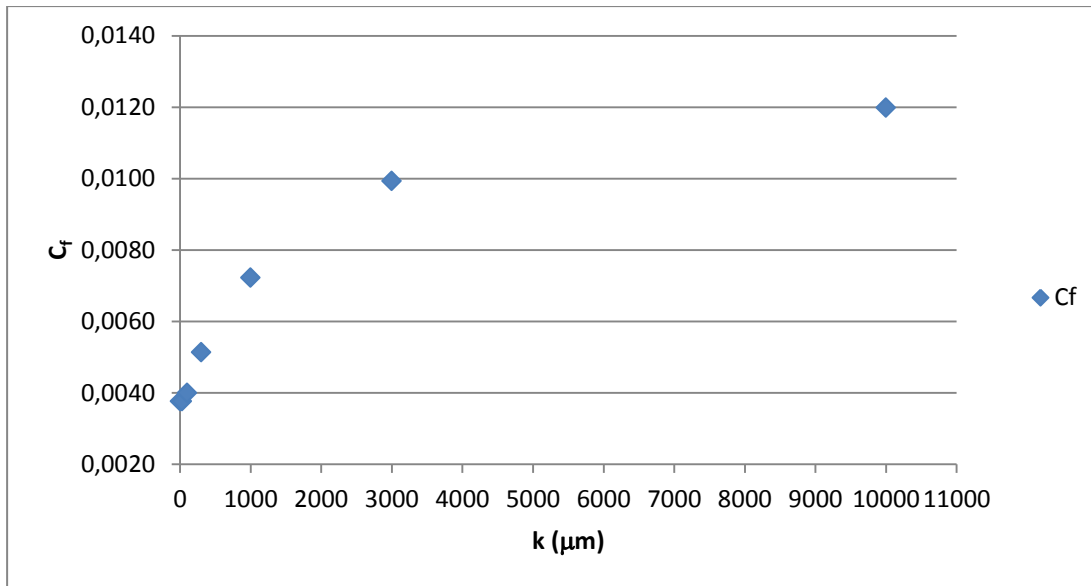
Şekil 5.32 : Bir dizi temsili boya ve fouling durumu için bulunan sürtünme direnci katsayılarının pürüzlülük yüksekliğine göre değişimi.
