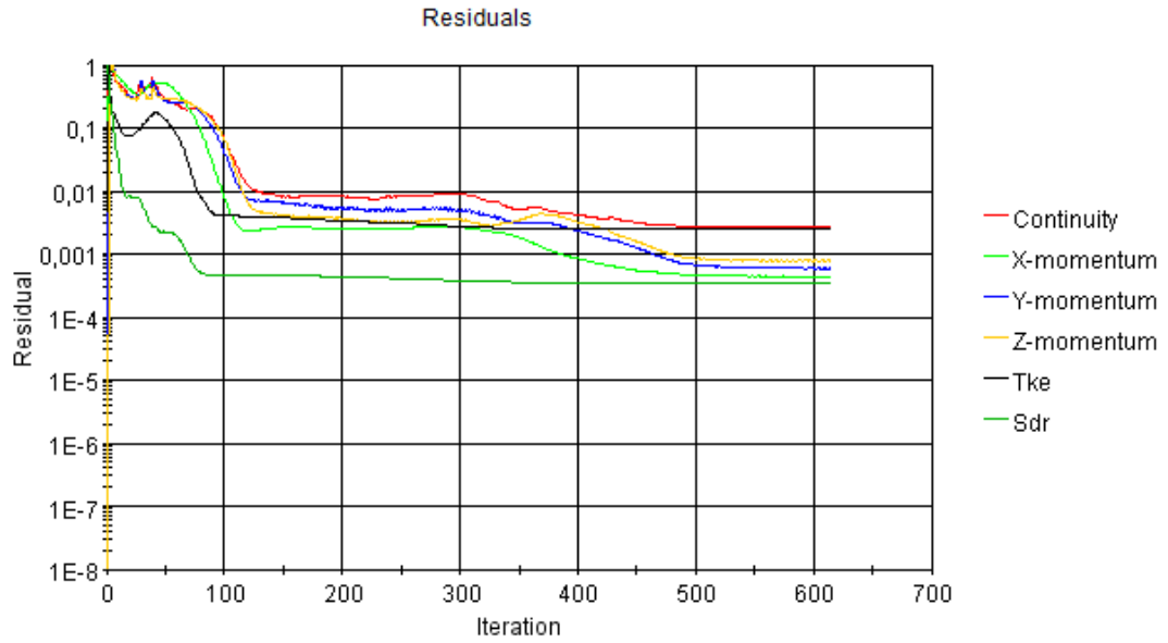
Şekil 5.26 : 220 numara zımpara kağıdı ile sarılmış plakanın analiz artık sonuçları iterasyonları.
