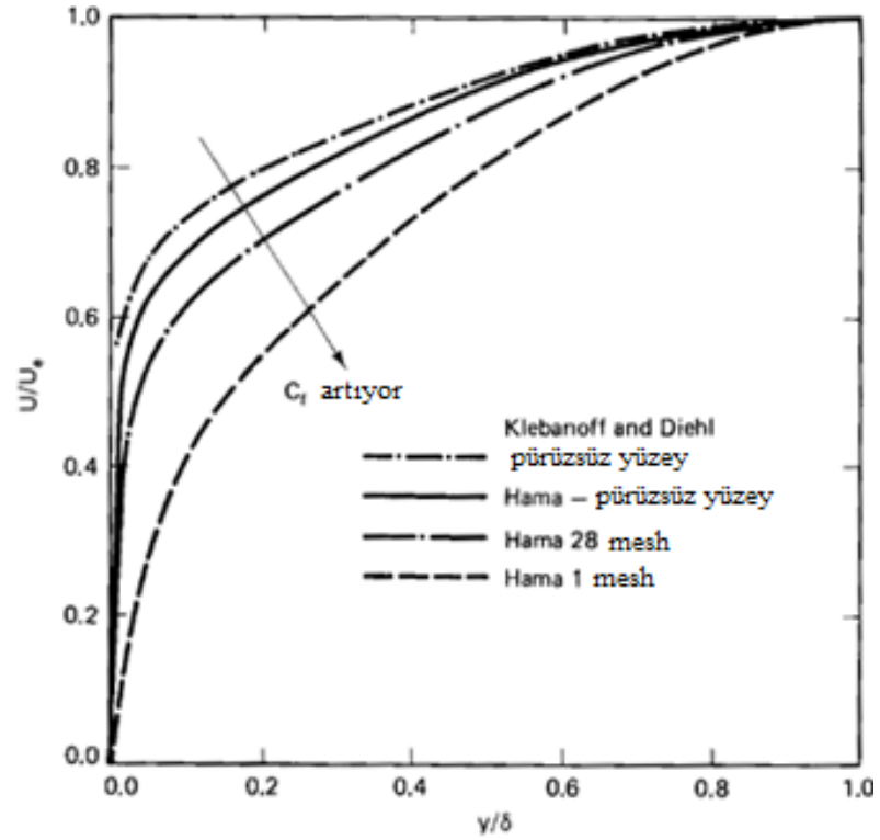
Şekil 4.9 : Pürüzsüz ve pürüzlü düz plakalar üzerindeki türbülans sınır tabaka hız profilleri (Schetz, 1993).
