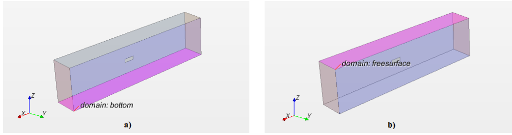
Şekil 5.6 : Çözüm hacminde a) dip ve b) serbest su yüzeyi.
