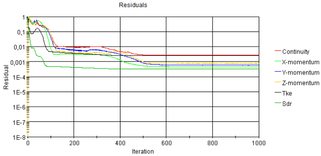
Şekil A. 27 : Pürüzlülük değeri k= 550 \mu m olan plakanın analiz artık sonuçları iterasyonları.
