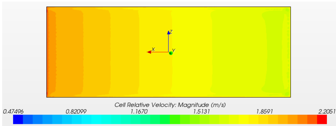
Şekil 5.42 : Global renk skalasına göre bozulmuş boya durumu veya hafif kaygan çamur tabakası oluşumu durumunda yüzey yerel akış hızları.
