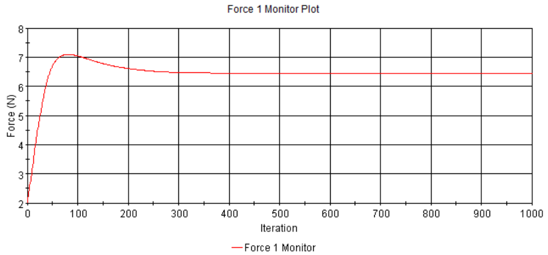
Şekil B. 2 : Pürüzlülük değeri k = 30 \mu m olan plakanın sürtünme direnci iterasyonları.
