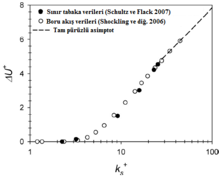
Şekil 4.16 : Pürüzlülük fonksiyonu ve pürüzlülük Reynolds sayısı arasındaki ilişki (Schultz ve Flack, 2007).
