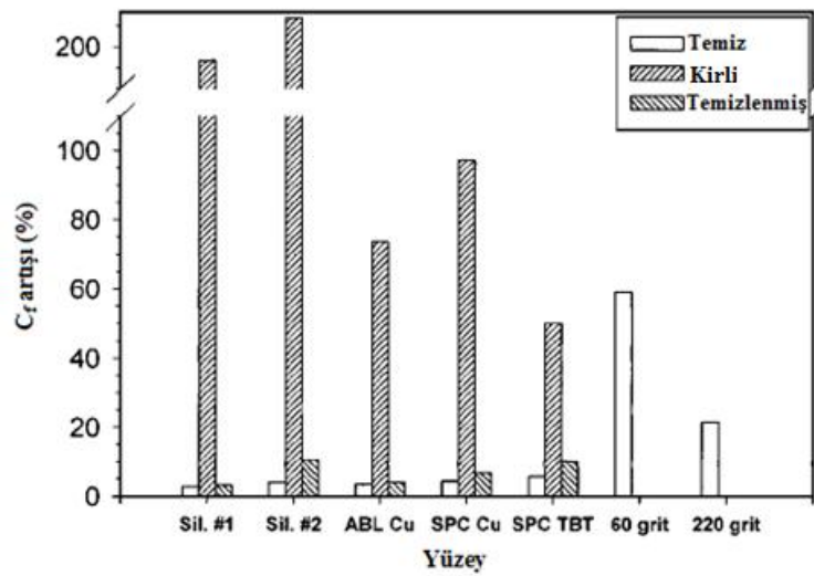
Şekil 4.30 : 12 knot hızında temiz, fouling 'emaruz kalmış ve temizlenmiş durumlar için gemi boyutundaki (L=150m.) sürtünme direnci katsayısı artışı tahmini (Schultz, 2004).
