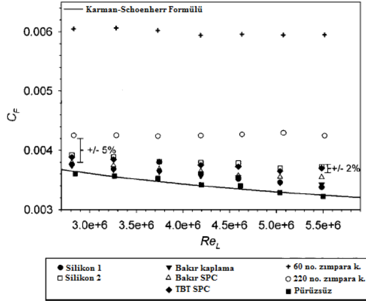
Şekil 4.29 : Temizlenmiş plakaların farklı Reynolds sayıları için bulunan sürtünme direnci katsayıları (Schultz, 2004).
