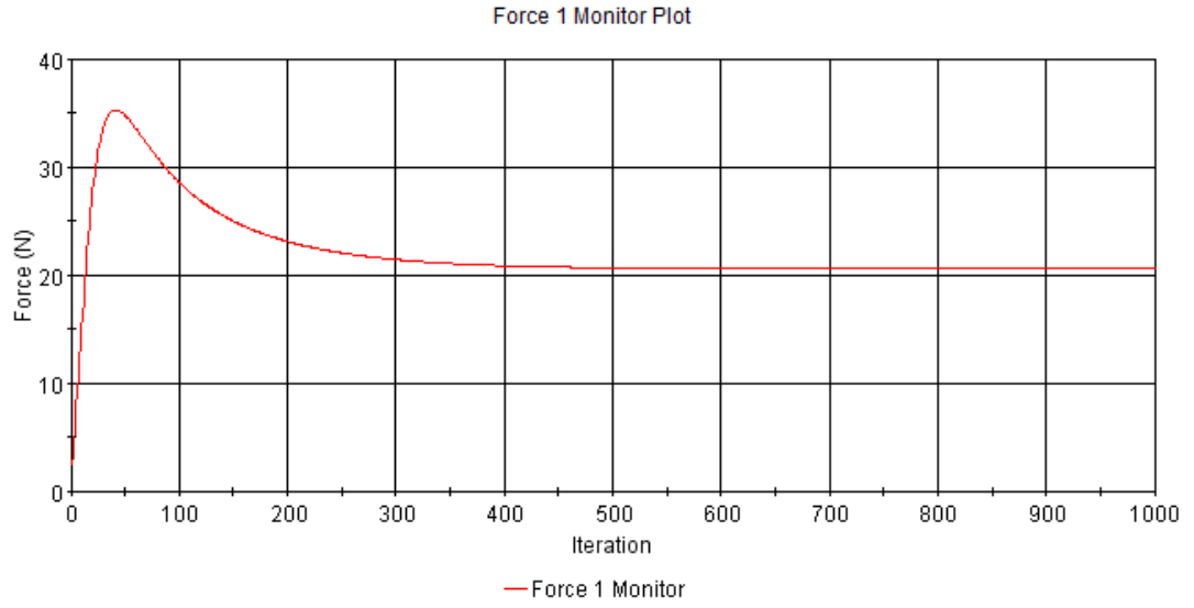
Şekil B. 17 : Pürüzlülük değeri k = 10000 \mu m olan plakanın sürtünme direnci iterasyonları.
