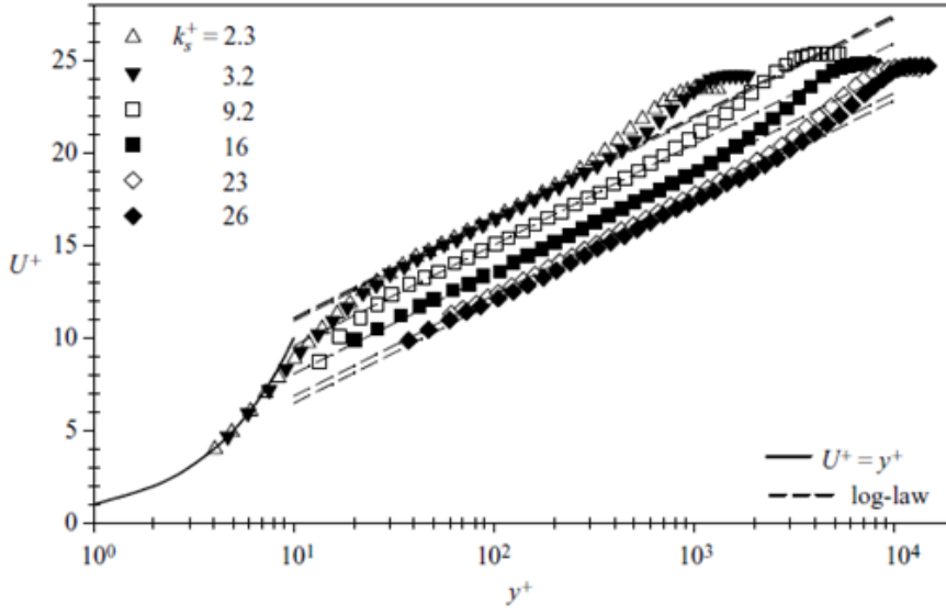
Şekil 4.15 : Pürüzlülük Reynold sayısındaki artışın hız profili üzerindeki etkileri (Schultz ve Flack, 2007).
