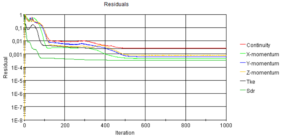
Şekil B. 9 : Pürüzlülük değeri k = 300 \mu m olan plakanın analiz artık sonuçları iterasyonları.
