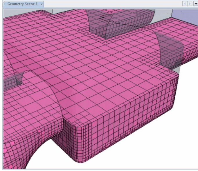
Şekil 5.14 : Trimmer hücreler ile örülen bir ağ örneği (CD-ADAPCO, 2011).
