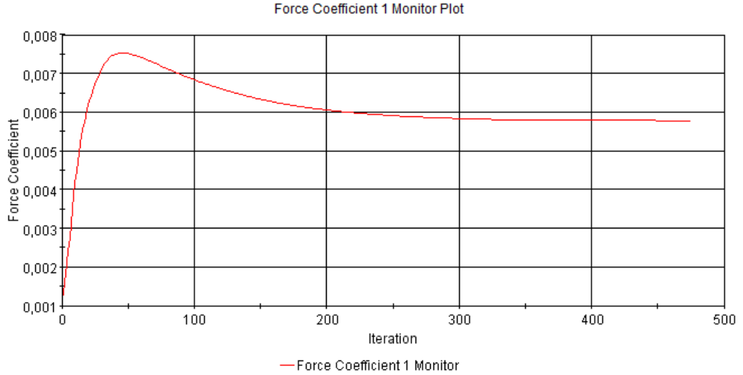
Şekil 5.21 : 60 numara zımpara kağıdı ile sarılmış plakanın sürtünme direnci katsayısı iterasyonları.
