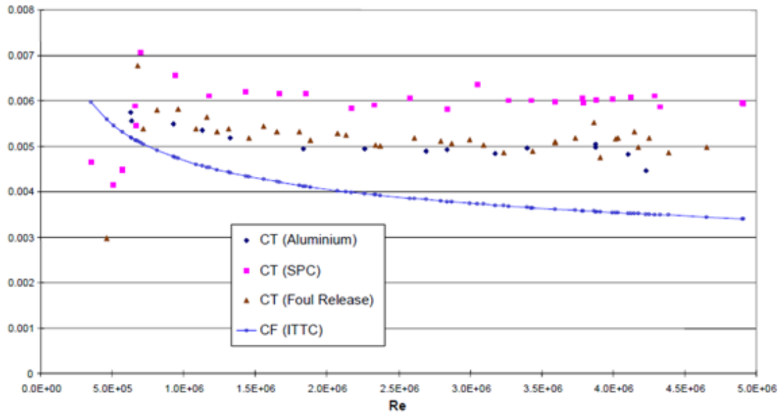
Şekil 4.24 : Farklı Reynolds sayıları için bulunan toplam direnç katsayıları (Candries, 2001).
