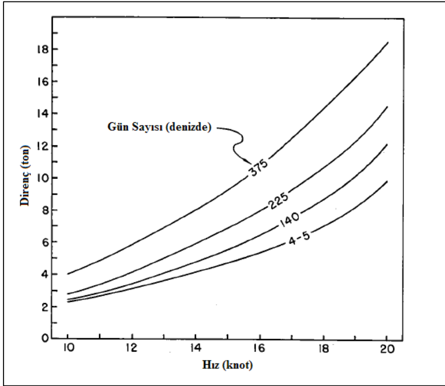
Şekil 4.21 : Yudachi destroyerinin havuzlamadan sonra farklı hızlarla yapılan çekme deneylerindeki direnç değerleri (Izubuchi, 1934).
