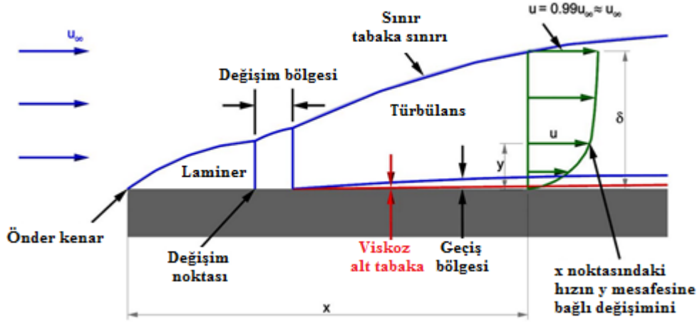
Şekil 4.7 : Düz bir plaka üzerinde oluşan türbülans sınır tabaka (Url-7).
