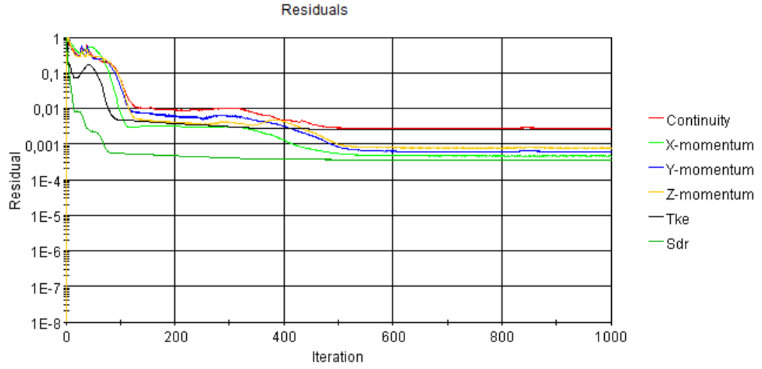
Şekil A. 33 : Pürüzlülük değeri k = 650 \mu m olan plakanın analiz artık sonuçları iterasyonları.
