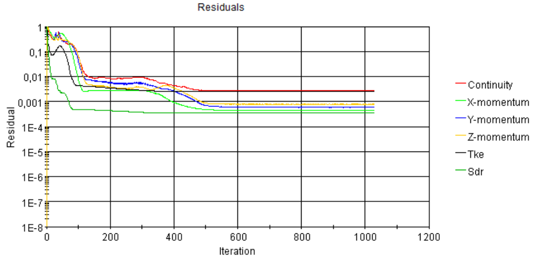
Şekil A. 9 : Pürüzlülük değeri k= 250 \mu m olan plakanın analiz artık sonuçları iterasyonları.
