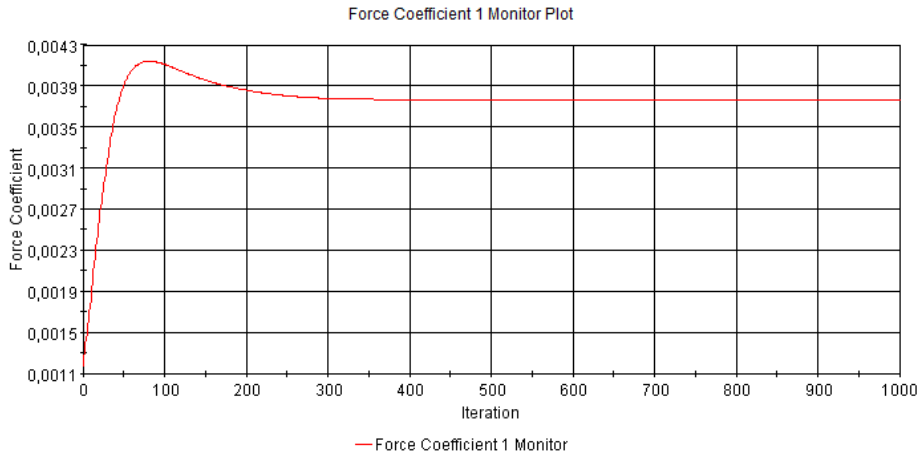
Şekil 5.18 : Pürüzsüz plakanın sürtünme direnci katsayısı iterasyonları.
