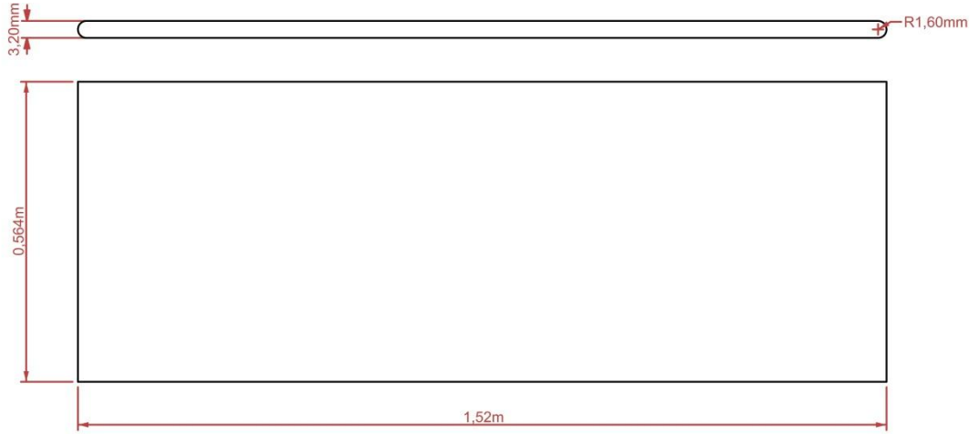
Şekil 5.1 : Plakanın ana boyutları.
