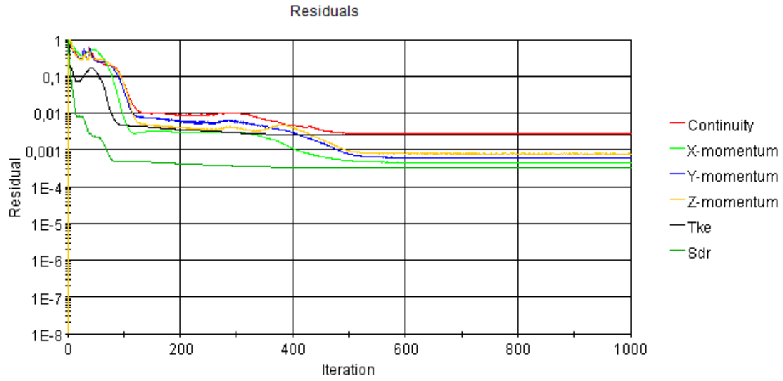
Şekil A. 15 : Pürüzlülük değeri k= 350 \mu m olan plakanın analiz artık sonuçları iterasyonları.
