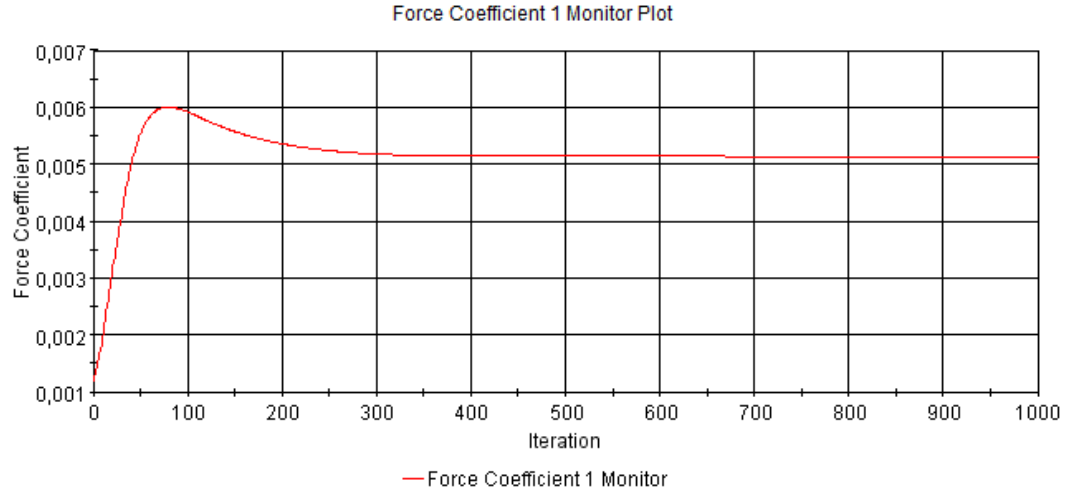
Şekil A. 10 : Pürüzlülük değeri k= 300 \mu m olan plakanın sürtünme direnci katsayısı iterasyonları.
