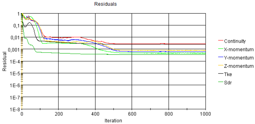
Şekil A. 36 : Pürüzlülük değeri k = 700 \mu m olan plakanın analiz artık sonuçları iterasyonları.
