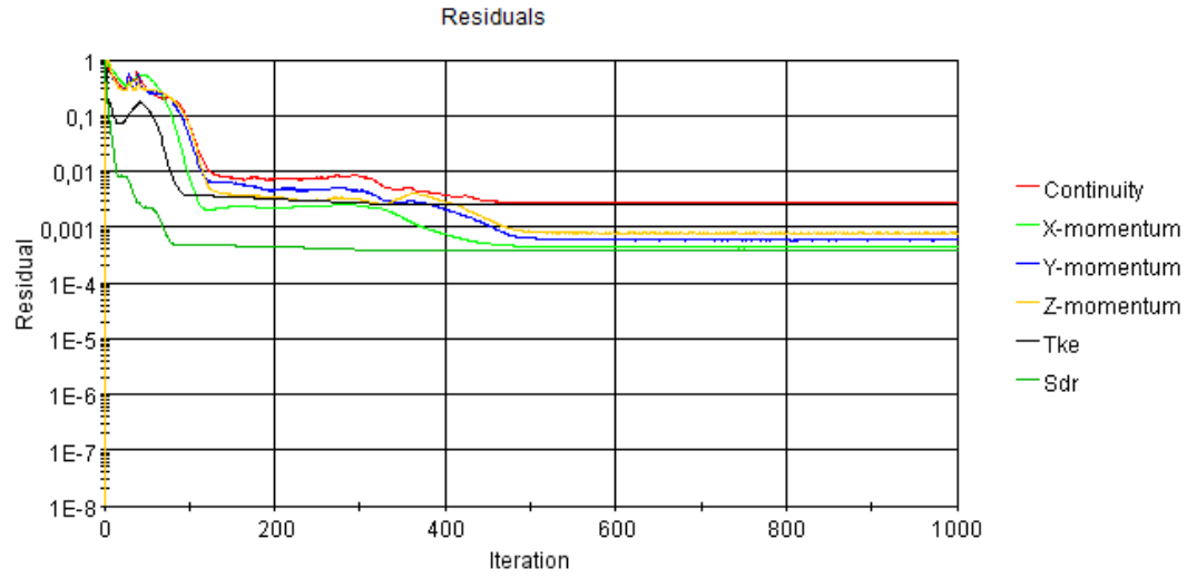
Şekil A. 3 : Pürüzlülük değeri k=100 \mu m olan plakanın analiz artık sonuçları iterasyonları.
