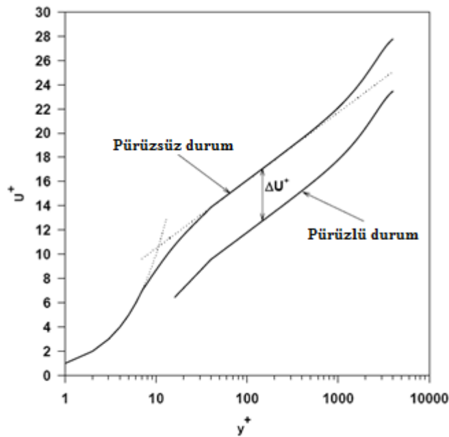
Şekil 4.14 : Pürüzlülüğün duvar kanununa etkisi (Schultz ve Swain, 2000).
