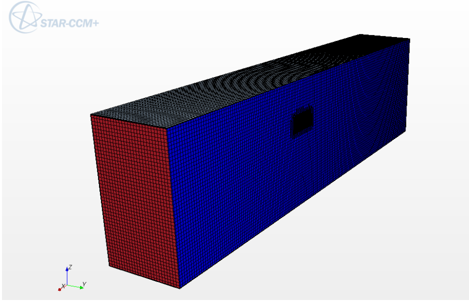
Şekil 5.10 : Çözüm ağı.
