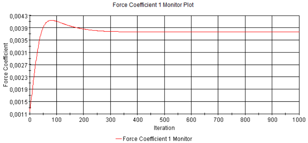
Şekil B. 1 : Pürüzlülük değeri k = 30 \mu m olan plakanın sürtünme direnci katsayısı iterasyonları.
