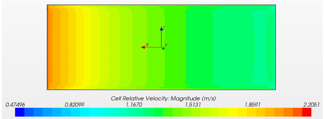
Şekil 5.45 : Global renk skalasına göre orta kalkerli fouling durumunda yüzey yerel akış hızları.
