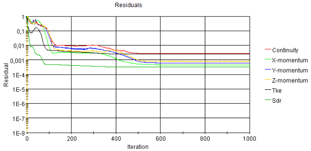
Şekil A. 18 : Pürüzlülük değeri k= 400 \mu m olan plakanın analiz artık sonuçları iterasyonları.
