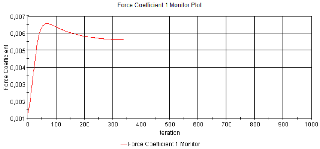
Şekil A. 19 : Pürüzlülük değeri k= 450 \mu m olan plakanın sürtünme direnci katsayısı iterasyonları.
