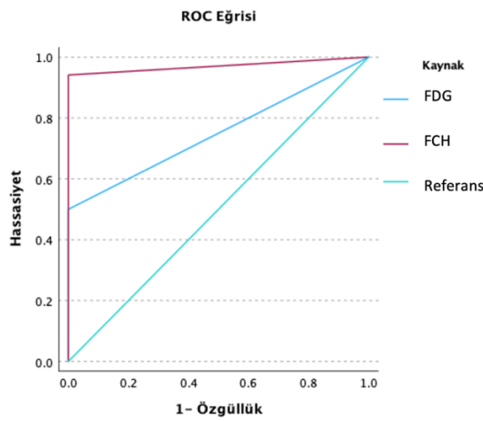
Şekil 4.13 ROC Analizi
