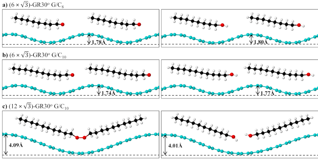
Şekil 5.3: Serbest grafen üzerinde alkantiyol ( G/C_n ) çizgili fazlı adsorpsiyon yapılarının optimize edilmiş geometrileri. (6 \times \sqrt{3}) -GR30° hücresinde (altın alttaş silinmiş olarak) grafen üzerindeki kemisorbe (solda) ve fizisorbe (sağda) a) oktantiyol ve b) dekantiyol çizgili faz yapıları, c) (12 \times \sqrt{3}) -GR30° hücresinde (altın alttaş silinmiş olarak) grafen üzerindeki kemisorbe (solda) ve fizisorbe (sağda) dekantiyol çizgili faz yapıları. Faz yapılarının karşılaştırılması için, a) ve b) panellerinde (6 \times \sqrt{3}) -GR30° periyodikliği iki kez tekrarlanmıştır.
