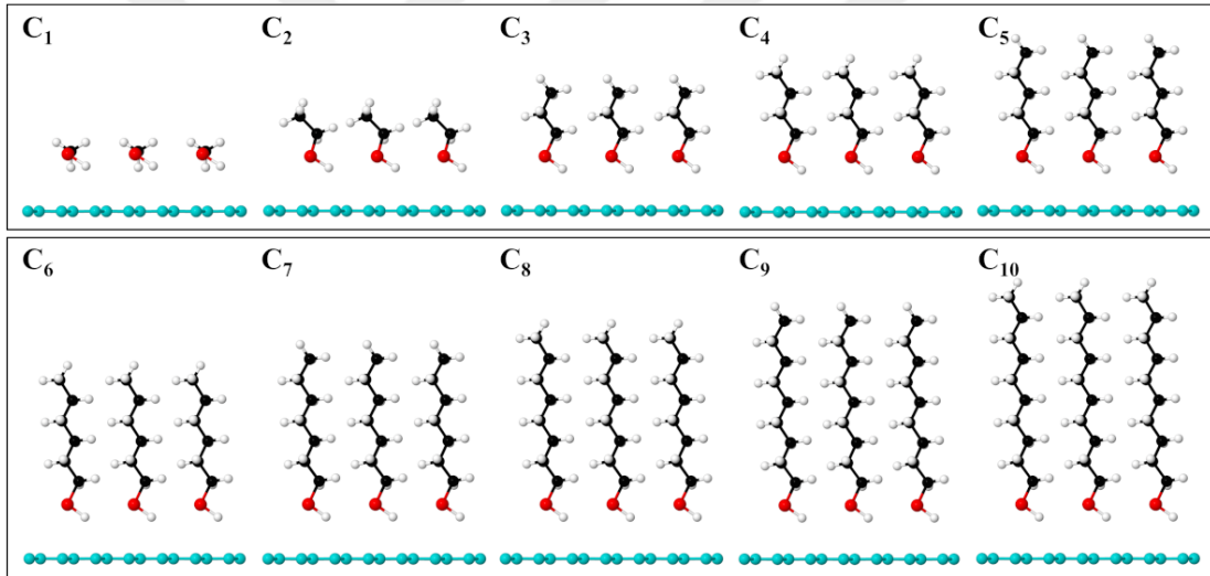
Şekil 6.5: (\sqrt{3} \times \sqrt{3})R30^\circ -GR30° Au(111)/G ortak süper hücresinde altın levha silindikten sonra kalan temiz grafen tabakası üzerinde dik fazlı fizisorbe alkantiyol yapısının (G/C n ) vdW-DFT yöntemiyle optimize edilmiş geometrilerinin yandan görüntüleri.
