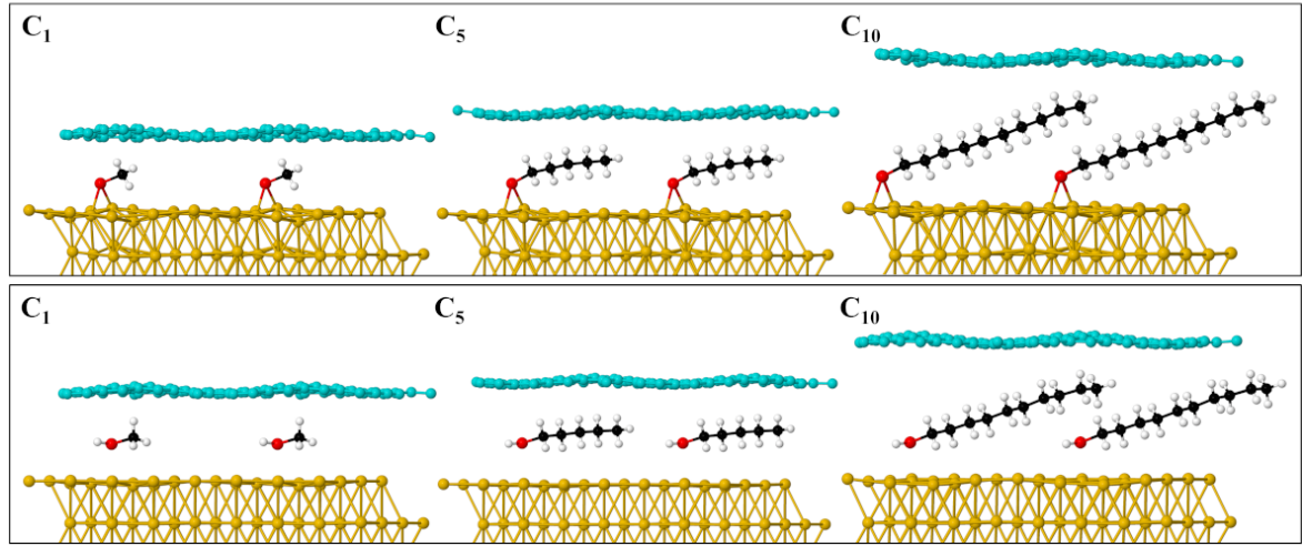
Şekil 6.22: (4 × 4)-GR10° hücresinde Au(111)/C n /G konformasyonu ile arayüzdeki yoğun fazlı kemisorbe (üst panel) ve fizisorbe (alt panel) alkantiyollerin optimize edilen geometrilerinin yandan görüntüleri. Alkantiyol yoğunluğunu göstermek için yüzey hücresi yanal yönde iki kez tekrarlanmıştır.
