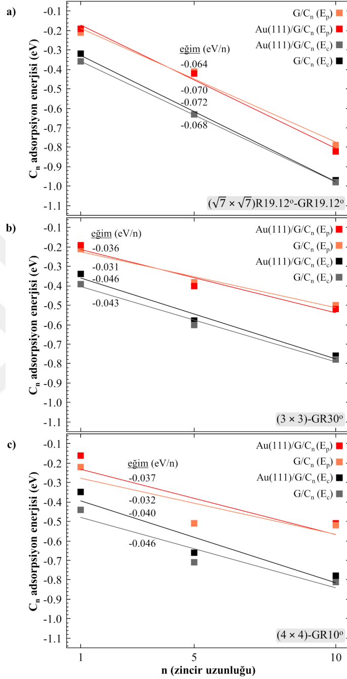
Şekil 6.19: a) (\sqrt{7} \times \sqrt{7})\text{R}19.12^\circ\text{-GR}19.12^\circ , b) (3 \times 3)\text{-GR}30^\circ ve c) (4 \times 4)\text{-GR}10^\circ hücreli Au(111)/G/C n ve G/C n konformasyonlarındaki yoğun fazlı alkantiyollerin adsorpsiyon enerjilerinin (E p : fizisorpsiyon, E c : kemisorpsiyon) zincir uzunluğuna göre değişimi ve doğrusal regresyonla belirlenen eğimleri (eV/n).
