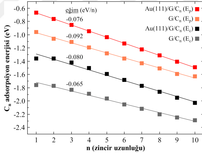
Şekil 4.5: (7 \times 7) -GR19.12° Au(111)/G ortak süper hücreli Au(111)/G/ C_n ve G/C_n konformasyonlarındaki alkantiyollerin adsorpsiyon enerjilerinin ( E_p : fizisorpsiyon, E_c : kemisorpsiyon) zincir uzunluğuna göre değişimi ve doğrusal regresyon eğim değerleri (eV/n).
