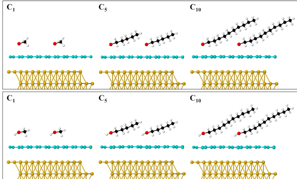
Şekil 6.14: (3 \times 3)\text{-GR}30^\circ \text{Au}(111)/\text{G} ortak süper hücresinde \text{Au}(111)/\text{G}/\text{C}_n ( n = 1, 5 ve 10 ) konformasyonu ile grafen tabakası üzerinde yoğun fazlı kemisorbe (üst panel) ve fizisorbe (alt panel) alkantiyollerin optimize edilen geometrilerinin yandan görüntüleri. Alkantiyol yoğunluğunu göstermek için yüzey hücresi yanal yönde iki kez tekrarlanmıştır.
