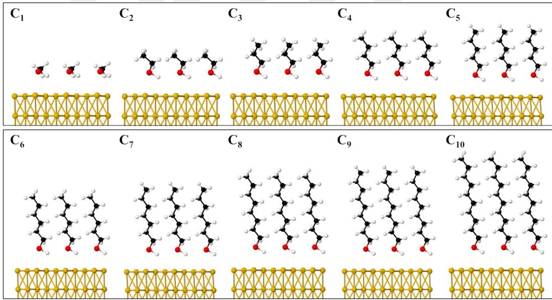
Şekil 6.10: Au(111)-( \sqrt{3} \times \sqrt{3} )R30° üzerinde dik fazlı alkantiyol fızisorpsiyon yapılarının optimize edilmiş geometrilerinin yandan görüntüleri.
