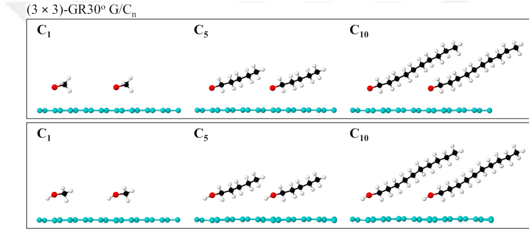
Şekil 6.17: (3 \times 3) -GR30° hücresinde altın levha silindikten sonra kalan temiz grafen üzerinde kemisorbe (üst panel) ve fizisorbe (alt panel) alkantiyol yapılarının (G/C n ) vdW-DFT yöntemiyle optimize edilmiş geometrilerinin yandan görüntüleri.
