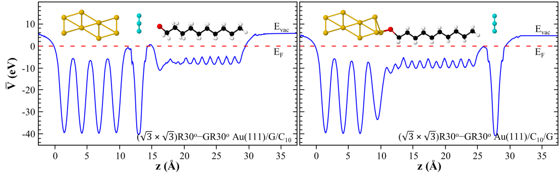
Şekil 6.12: (\sqrt{3} \times \sqrt{3})R30^\circ\text{-GR}30^\circ Au(111)/G ortak süper hücreli Au(111)/G/ C_n ve Au(111)/ C_n /G konformasyonlarında dik fazlı dekantiyol yapılarının planar ortalama elektrostatik potansiyel enerji profilleri. (z eksen [111] ile çakışmıştır.)
