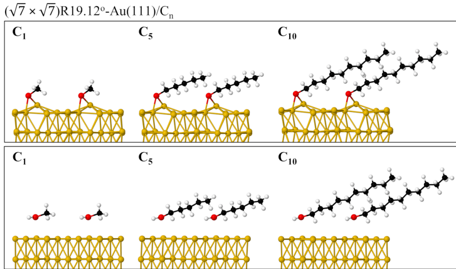
Şekil 6.23: Au(111)- (\sqrt{7} \times \sqrt{7}) R19.12° üzerinde yoğun fazlı alkantiyol kemisorpsiyon (üst panel) ve fizisorpsiyon (alt panel) yapılarının optimize edilmiş geometrilerinin yandan görüntüleri.
