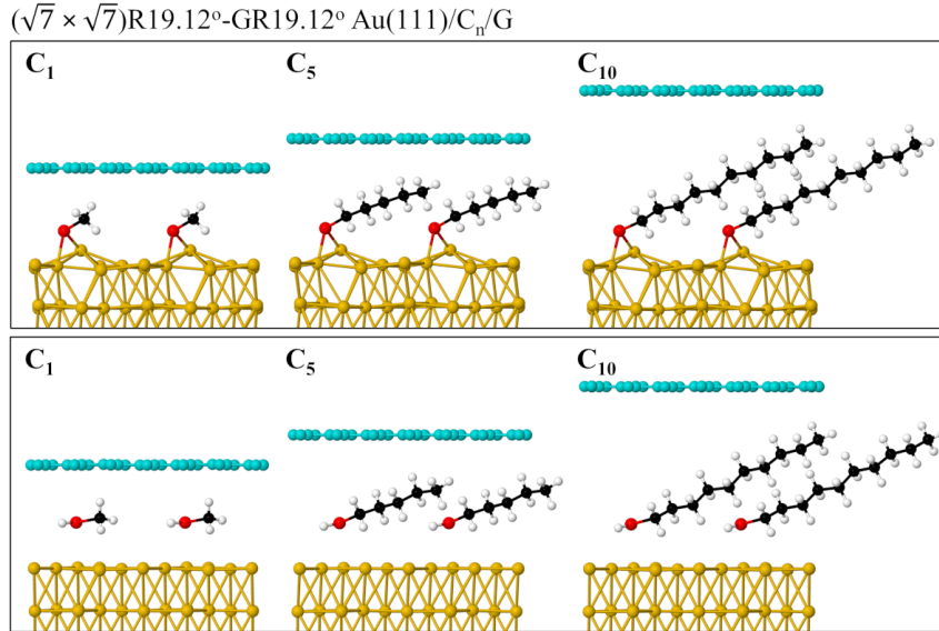
Şekil 6.20: (\sqrt{7} \times \sqrt{7})R19.12^\circ -GR19.12° hücresinde Au(111)/C n /G konformasyonu ile arayüzdeki yoğun fazlı kemisorbe (üst panel) ve fizisorbe (alt panel) alkantiyollerin optimize edilen geometrilerinin yandan görüntüleri. Alkantiyol yoğunluğunu göstermek için yüzey hücresi yanal yönde iki kez tekrarlanmıştır.
