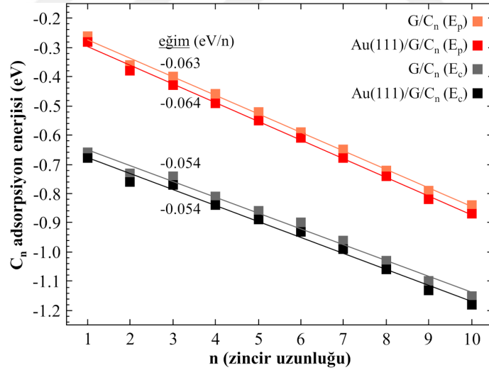
Şekil 6.6: (\sqrt{3} \times \sqrt{3})R30^\circ\text{-GR}30^\circ Au(111)/G ortak hücreli Au(111)/ G/C_n ve G/C_n yapılarında dik fazlı alkantiyollerin adsorpsiyon enerjilerinin ( E_p : fizisorpsiyon, E_c : kemisorpsiyon) zincir uzunluğuna göre değişimi ve doğrusal regresyon eğimleri (eV/n).
