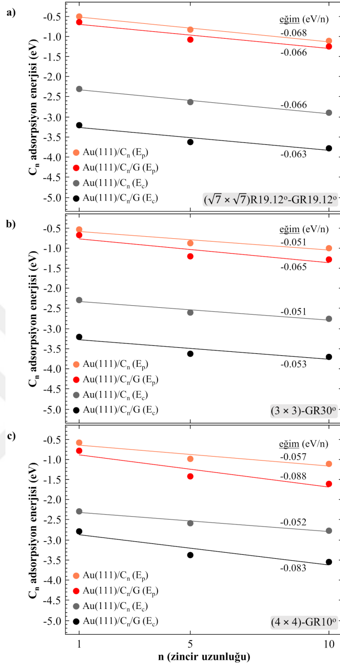
Şekil 6.26: a) (\sqrt{7} \times \sqrt{7})R19.12^\circ\text{-GR}19.12^\circ , b) (3 \times 3)\text{-GR}30^\circ ve c) (4 \times 4)\text{-GR}10^\circ ortak süper hücreli Au(111)/C n /G ve Au(111)/C n konformasyonlarında alkantiyollerin adsorpsiyon enerjilerinin (E p : fizisorpsiyon, E c : kemisorpsiyon) zincir uzunluğuna göre değişimi ve doğrusal regresyonla belirlenen eğimleri (eV/n).
