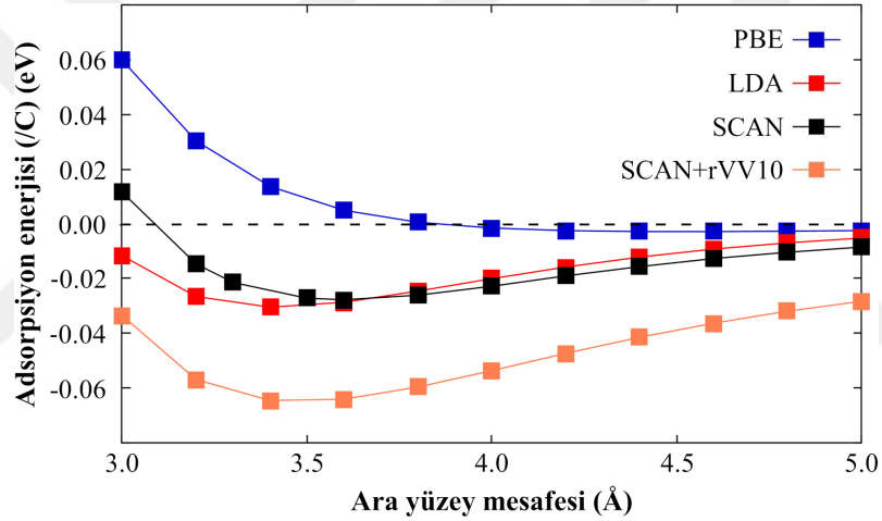
Şekil 3.3: Farklı değiş-tokuş ve korelasyon (XC) fonksiyonelleri ile hesaplanmış, Au(111) yüzeyinde tutunan grafen tabakasındaki karbon atomu sayısı başına ortalama adsorpsiyon enerjisinin Au(111)/G ara yüzey mesafesine göre değişim profilleri.
