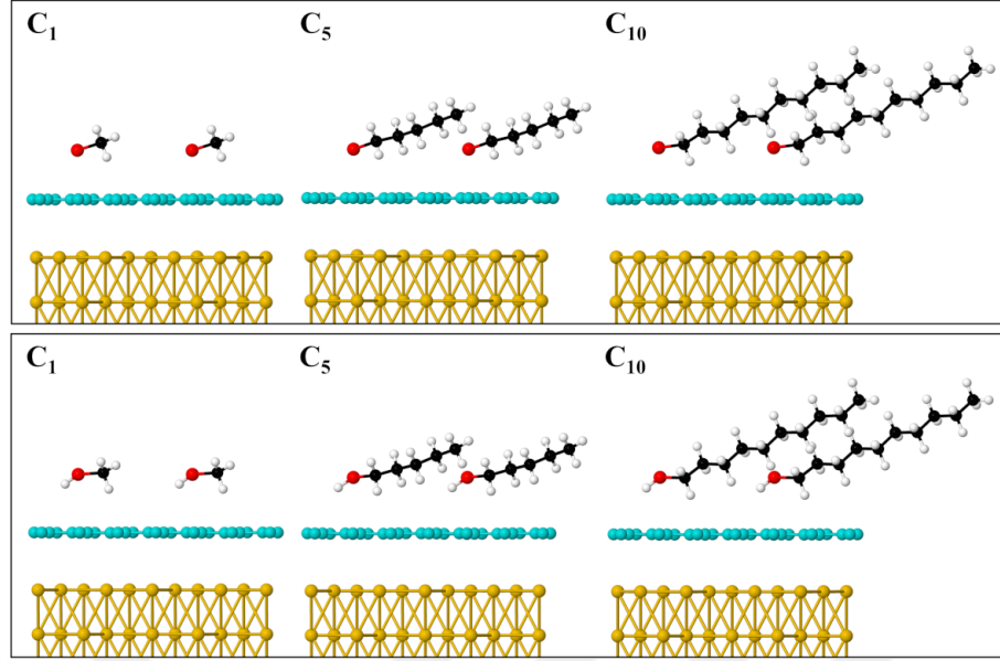
Şekil 6.13: (\sqrt{7} \times \sqrt{7})R19.12^\circ\text{-GR}19.12^\circ \text{Au}(111)/\text{G} ortak süper hücresinde \text{Au}(111)/\text{G}/\text{C}_n ( n = 1, 5 ve 10 ) konformasyonu ile grafen tabakası üzerinde yoğun fazlı kemisorbe (üst panel) ve fizisorbe (alt panel) alkantiyollerin optimize edilen geometrilerinin yandan görüntüleri. Alkantiyol yoğunluğunu göstermek için yüzey hücresi yanal yönde iki kez tekrarlanmıştır.
