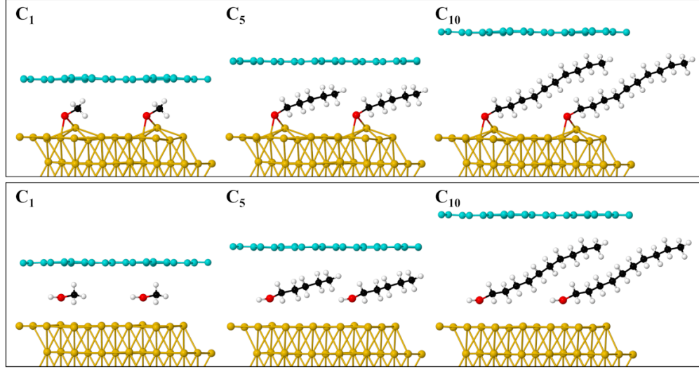
Şekil 6.21: (3 × 3)-GR30° hücresinde Au(111)/C n /G konformasyonu ile arayüzdeki yoğun fazlı kemisorbe (üst panel) ve fizisorbe (alt panel) alkantiyollerin optimize edilen geometrilerinin yandan görüntüleri. Alkantiyol yoğunluğunu göstermek için yüzey hücresi yanal yönde iki kez tekrarlanmıştır.
