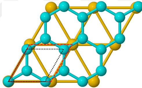
Şekil 3.1: (2 × 2)-Au(111) yüzey tabakası üzerinde grafenin şematik gösterimi. Nuktalı (siyah) ve kesikli (kırmızı) çizgiler, sırasıyla grafen ve Au(111) birim hücrelerini göstermektedir.
