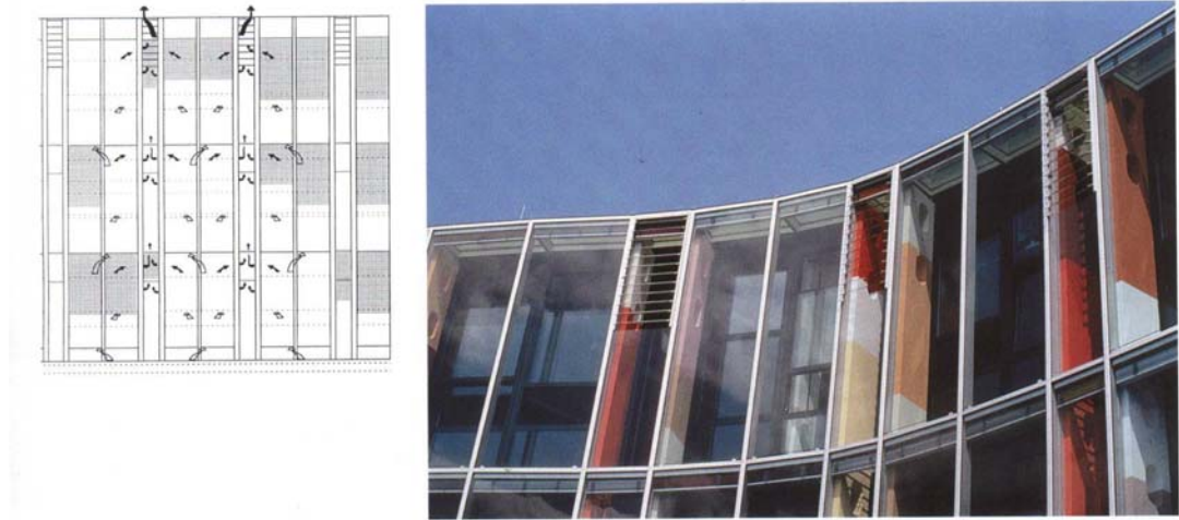
Şekil 2.45: Bir şaft tipi çift kabuklu cephede, kullanılmış havanın şafta girerek bunun içinden yükselmesi sonucunda üst kısımdan dış ortama atılması
