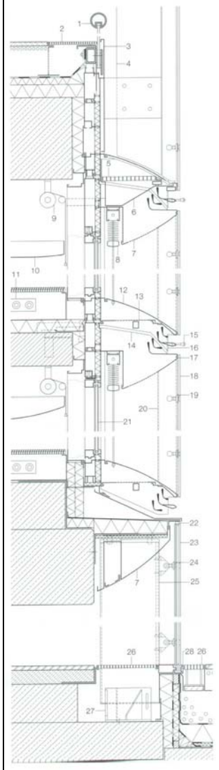
Şekil A.17: RWE Cephe Kesiti
