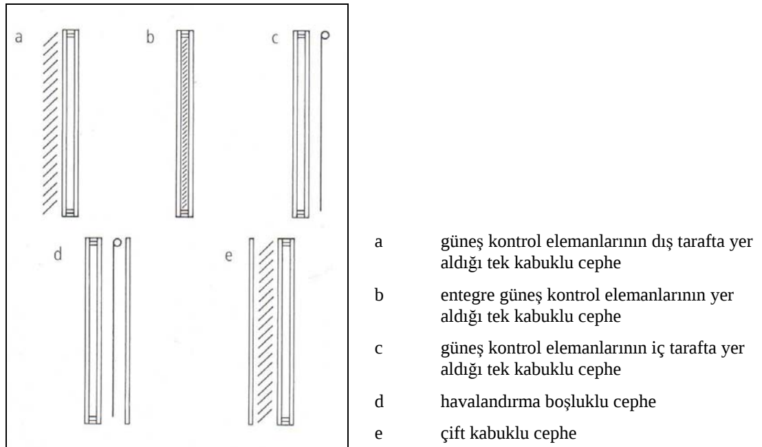
Şekil 2.5: Çok farklı türleri olan cam cephe sistemlerinin beş ana kategoride sınıflandırılması (Compagno, 2002, s.93)
