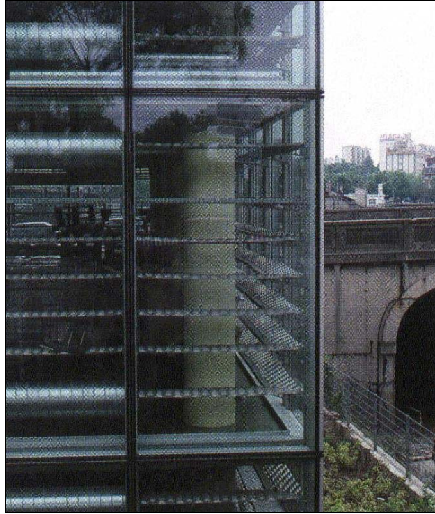
Şekil 2.20: Güneş kontrolünün iç taraftan; yatay lameller, açık kablo yolları ve havalandırma kanalları ile sağlanması
