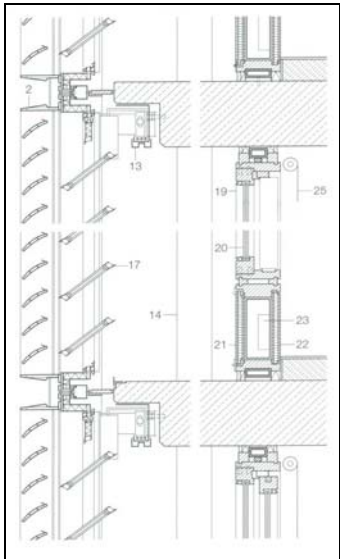
Şekil A.15: Messehochhaus 2.Cephe Kesiti
