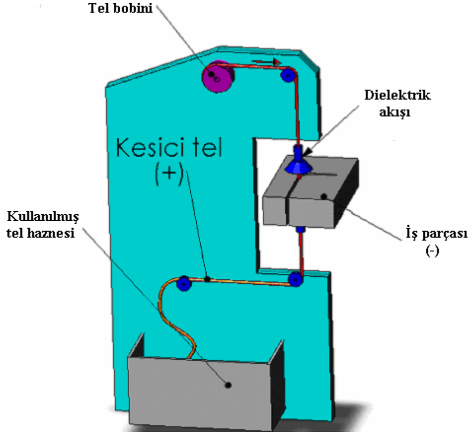
Şekil 3.1. Tel erozyon tezgahının(WEDM) işleme mantığı
