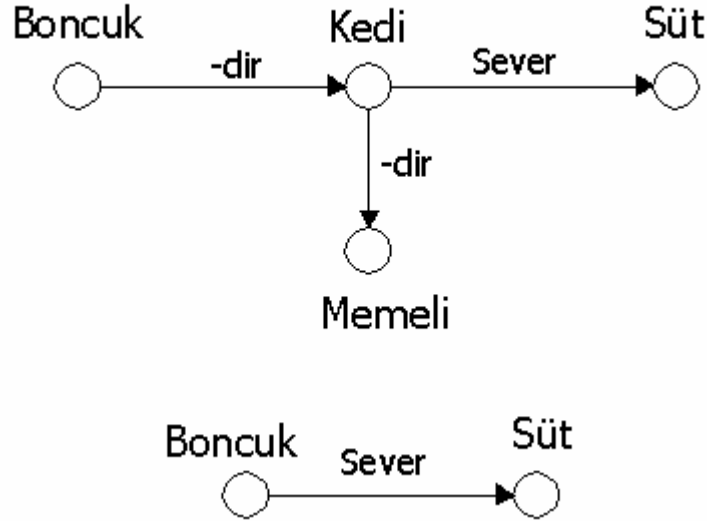
Şekil 2.3. Semantik şebeke yardımı ile çıkarım 1
