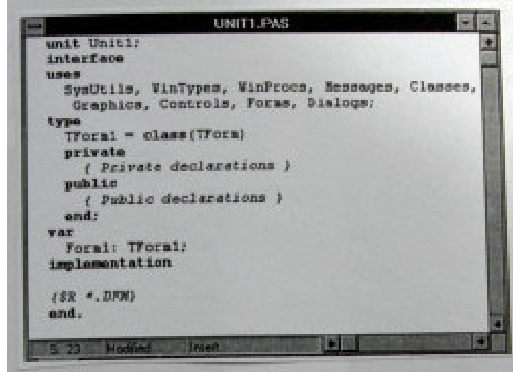
Şekil 3.6. UNIT1.PAS penceresi
