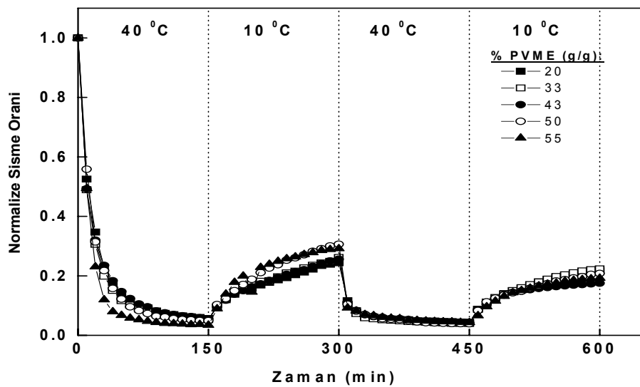
Şekil 4.7. P(TBAAm-ko-AAm)/PVME hidrojellerinin PVME miktarına bağlı 10 °C ve 40 °C' deki şişme-büzülme davranışları
