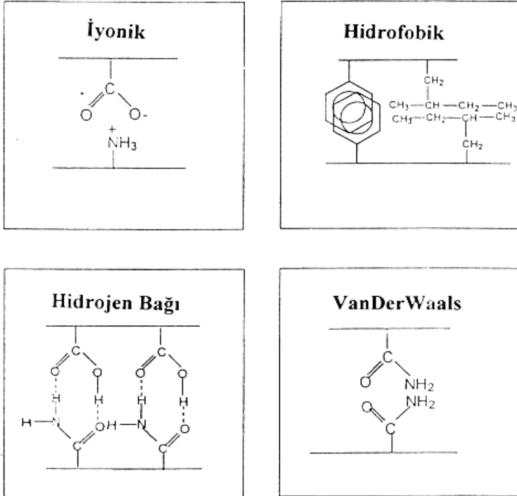
Şekil 2.5. Jellerin hacim faz geçişindeki temel etkileşimler
