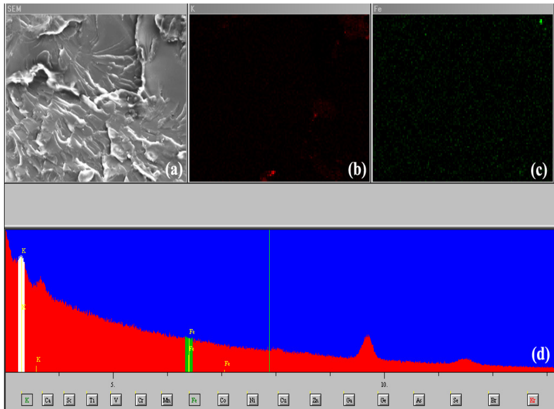
Resim 4.4. P(TBAAm-ko-AAm)/PVME hidrojjellerinin arayüzey SEM ve EDS görüntüleri (x 500)
