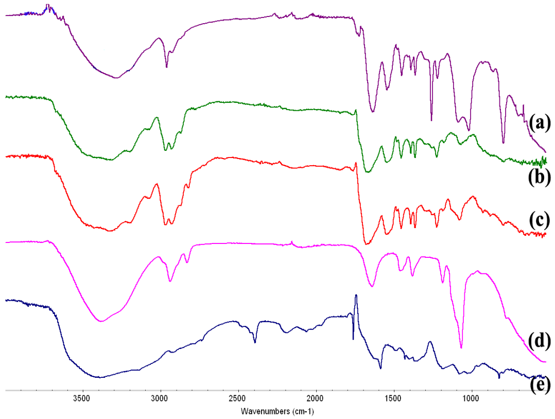
Şekil 4.14. P(TBAAm-ko-AAm)/PVME hidrojel ve ferrojelinin FT-IR spektrumu (a) P(TBAAm-ko-AAm)/PVME+Fe 3 O 4 :ferrojel, (b) P(TBAAm-ko-AAm)/PVME yarı-IPN hidroجلي, (c) P(TBAAm-ko-AAm) kopolimeri, (d) PVME polimeri, (e) magnetit : Fe 3 O 4
