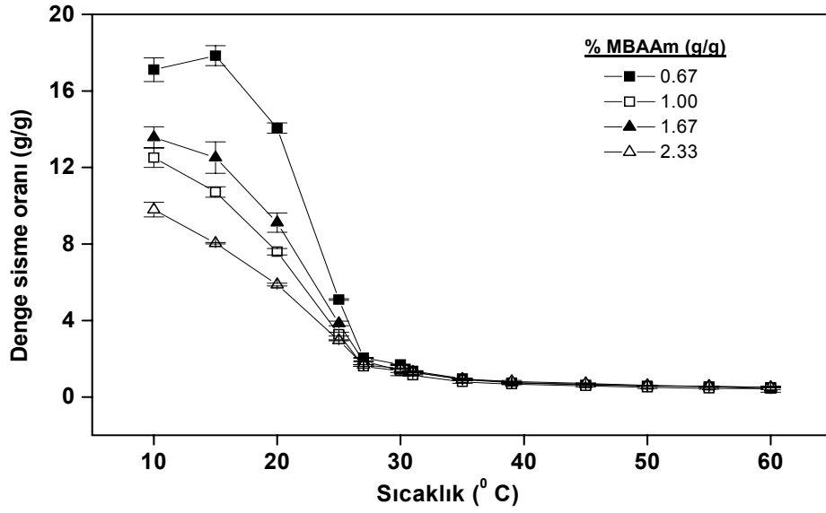
Şekil 4.4. P(TBAAm-ko-AAm)/PVME hidrojjellerinin çapraz bağlayıcı miktarına bağlı denge şişme oranı-sıcaklık eğrisi
