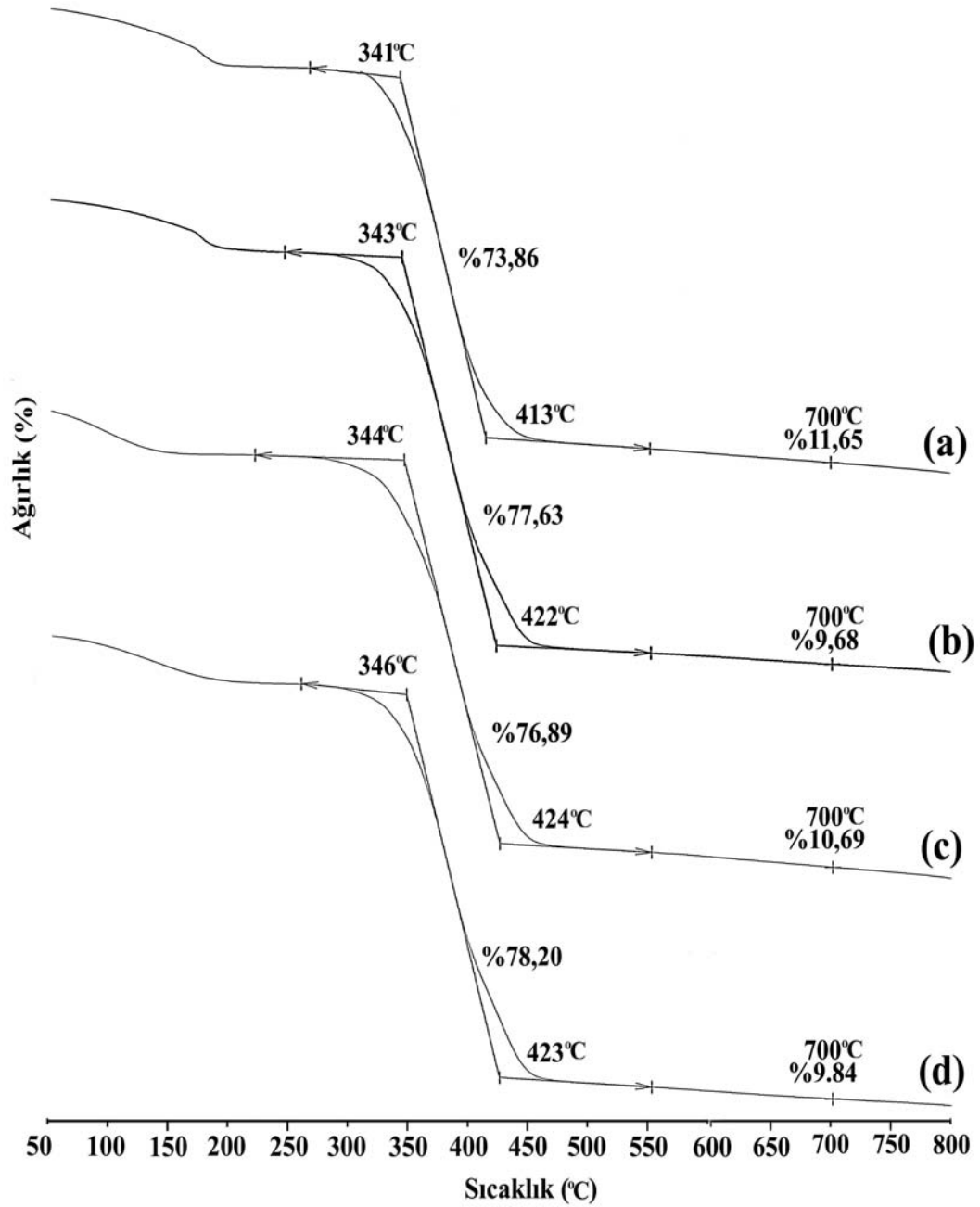
Şekil 4.10 Polimerizasyon yöntemi ile sentezlenmiş P(TBAAm-ko-AAm)/PVME ferrojellerine ait TGA termogramı; (a) % 20 PVME (b) % 33 PVME (c) % 43 PVME (d) % 50 PVME.
