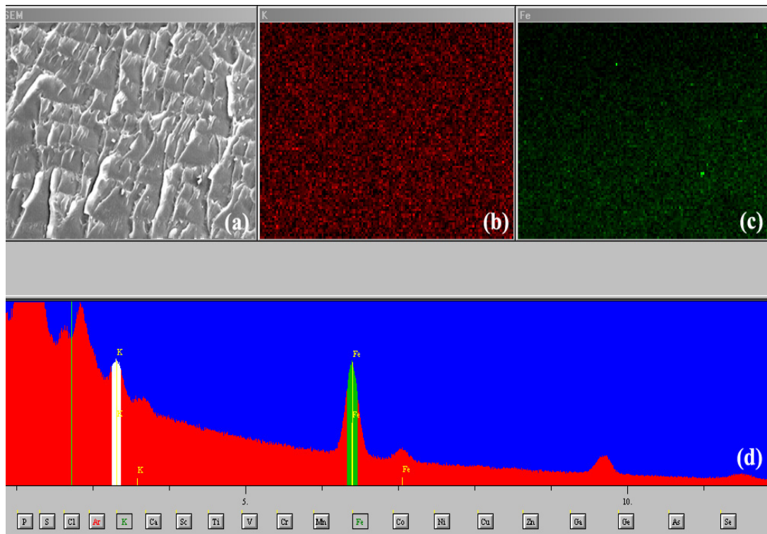
Resim 4.6. P(TBAAm-ko-AAm)/PVME ferrojellerinin arayüzey SEM ve EDS görüntüleri (x 500)
