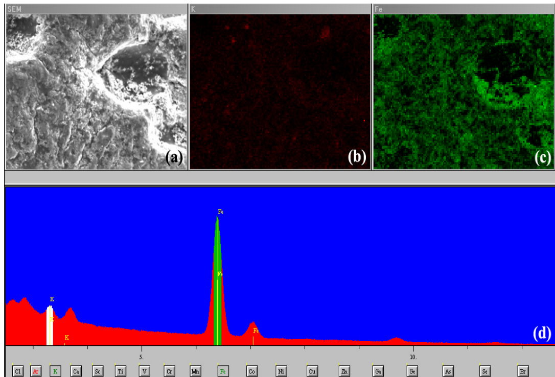
Resim 4.5. P(TBAAm-ko-AAm)/PVME ferrojellerinin yüzey SEM ve EDS görüntüleri (x 500)
