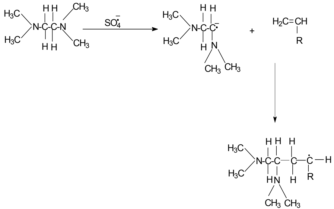
Şekil 4.1. APS ile TEMED reaksiyonu sonucunda oluşan ortaklanmamış elektron içeren aktif TEMED molekülünün monomere katılması
