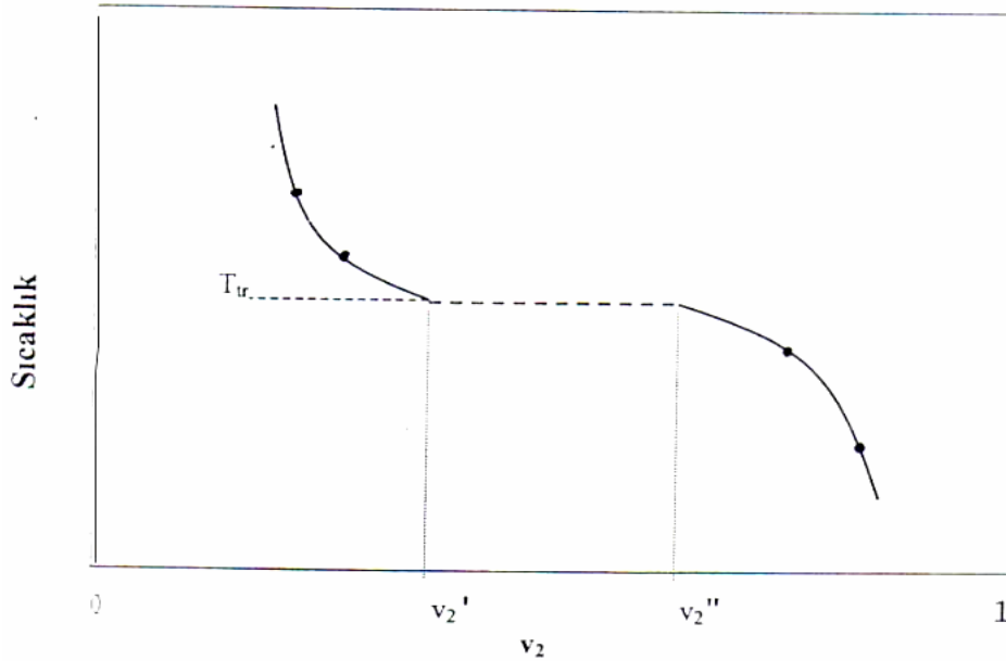
Şekil 2.4. Şişmiş bir jeldeki faz geçişini gösteren sıcaklık-hacim diyagramı
