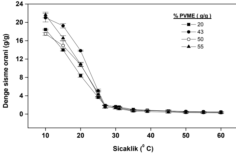
Şekil 4.6. P(TBAAm-ko-AAm)/PVME hidrojenlerinin PVME miktarına bağlı denge şişme oranı-sıcaklık eğrisi. (Polimerizasyon yöntemi ile hazırlanan).
