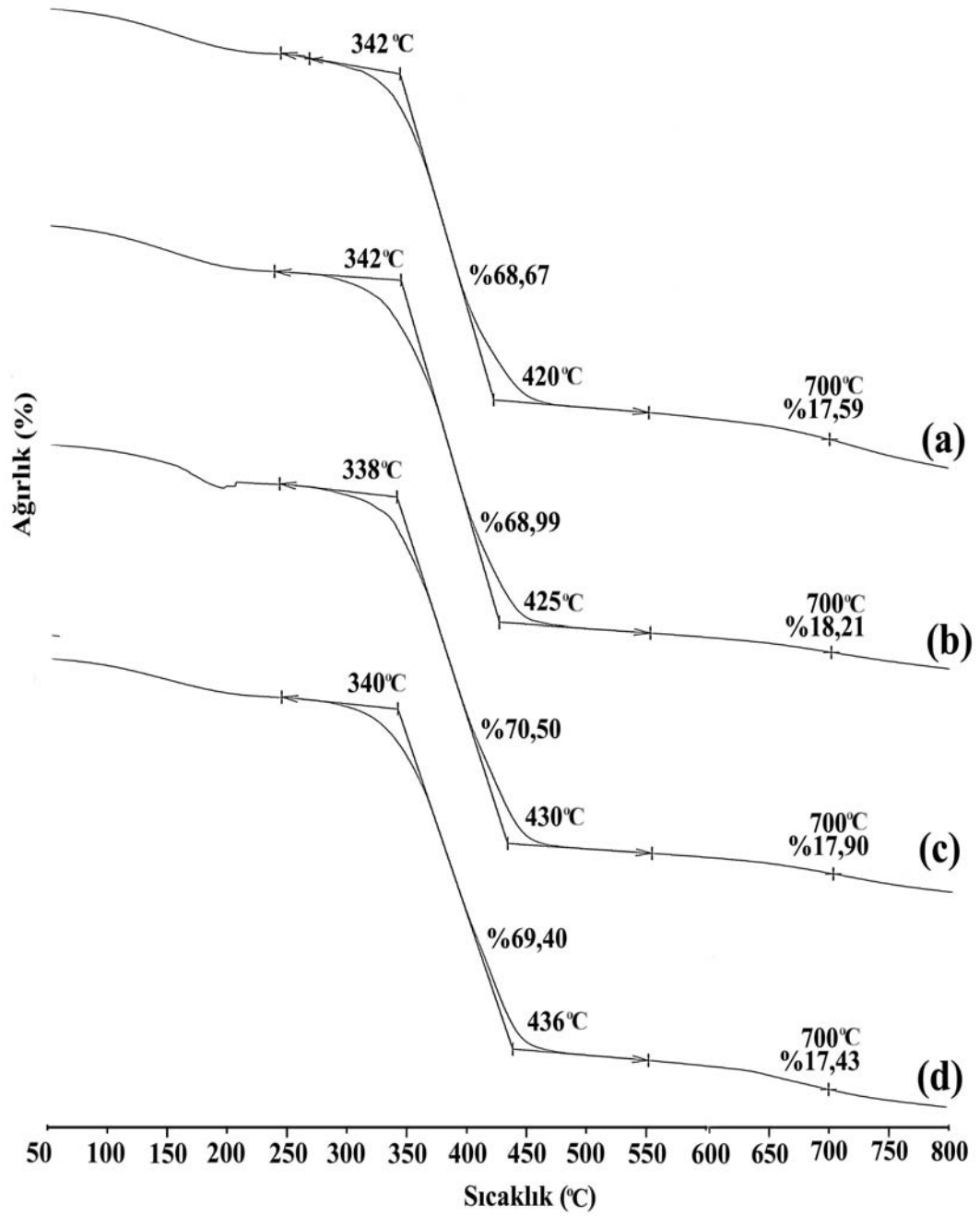
Şekil 4.11. Absorpsiyon yöntemi ile sentezlenmiş P(TBAAm-ko-AAm)/PMVE ferrojellerine ait TGA termogramı; (a) % 20 PVME (b) % 33 PVME (c) % 43 PVME (d) % 50 PVME.
