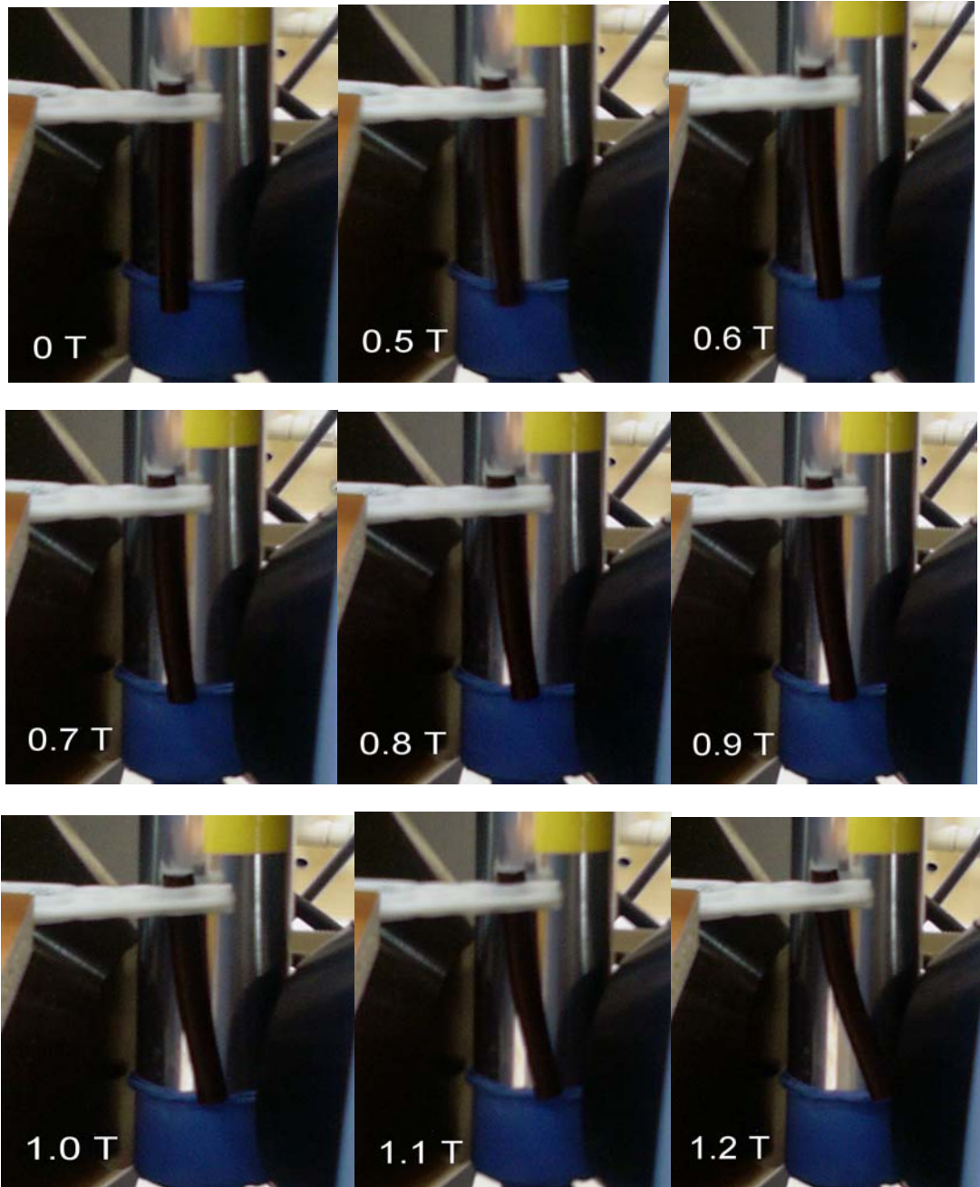
Resim 4.2. P(TBAAm-ko-AAm)/PVME ferrojellerinin manyetik alandaki şekil değişimi (absorpsiyon yöntemi ile hazırlanmış)
