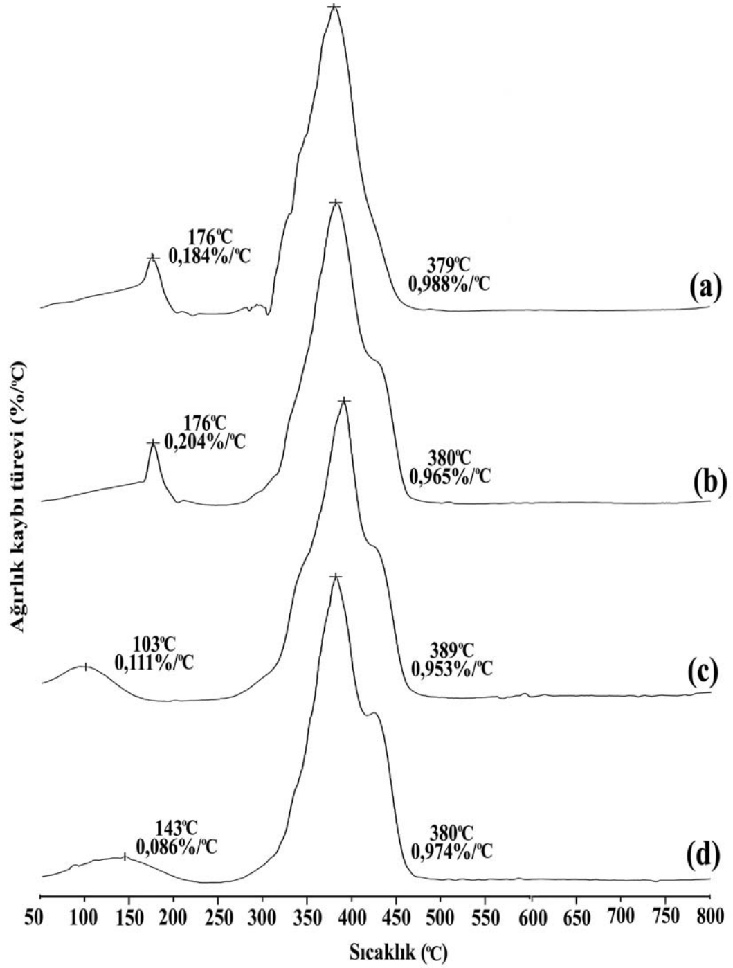
Şekil 4.12. Polimerizasyon yöntemi ile sentezlenmiş P(TBAAm-ko-AAm)/PVME ferrojellerine ait DTG termogramı; (a) % 20 PVME (b) % 33 PVME (c) % 43 PVME (d) % 50 PVME.
