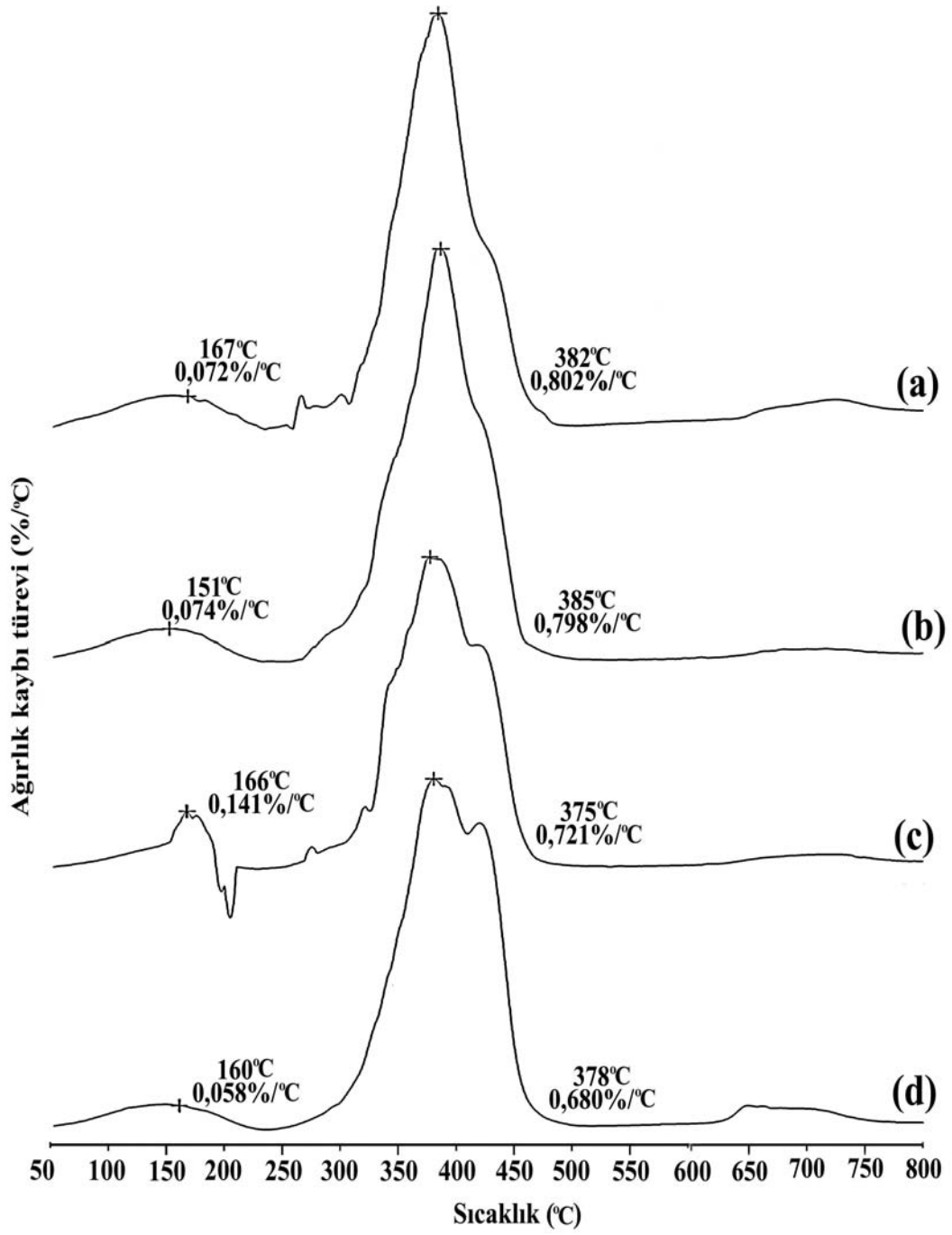
Şekil 4.13. Absorpsiyon yöntemi ile sentezlenmiş P(TBAAm-ko-AAm)/PMVE ferrojellerine ait DTG termogramı; (a) % 20 PVME (b) % 33 PVME (c) % 43 PVME (d) % 50 PVME.
