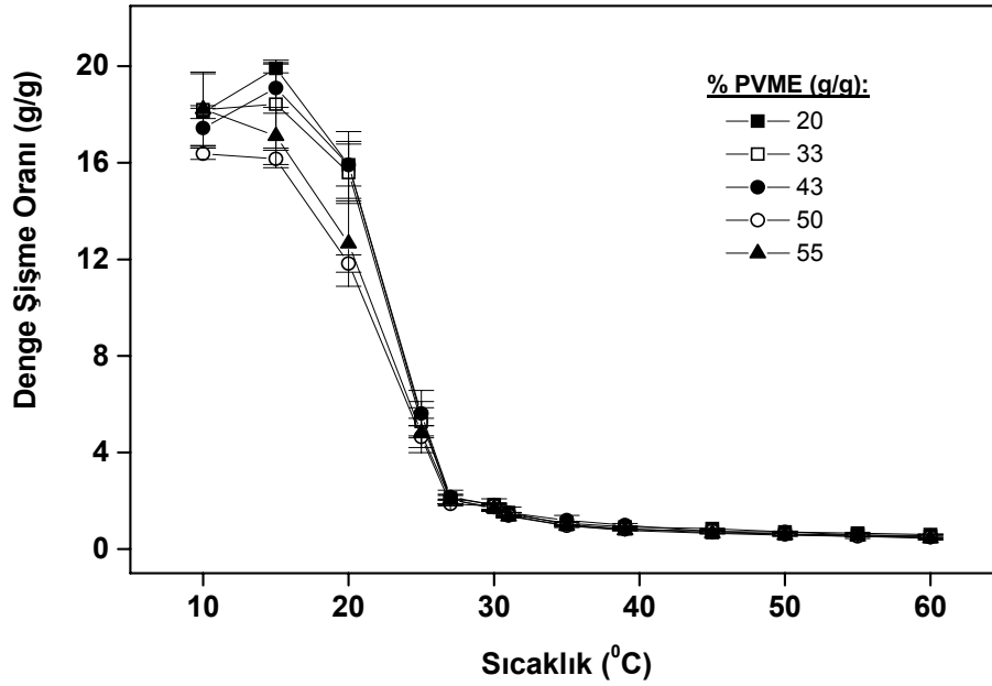
Şekil 4.5. P(TBAAm-ko-AAm)/PVME hidrojellerinin PVME miktarına bağlı denge şişme oranı-sıcaklık eğrisi (Absorpsiyon yöntemi ile hazırlanan)
