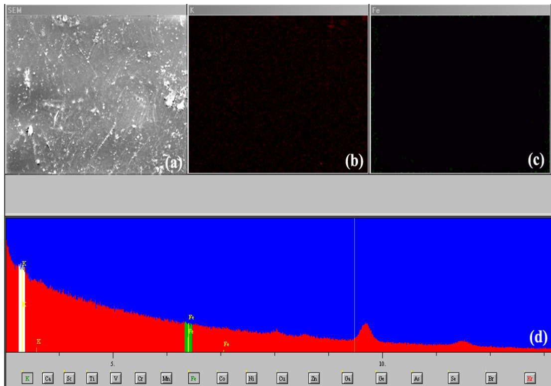
Resim 4.3. P(TBAAm-ko-AAm)/PVME hidrojellerinin yüzey SEM ve EDS görüntüleri (x 500)
