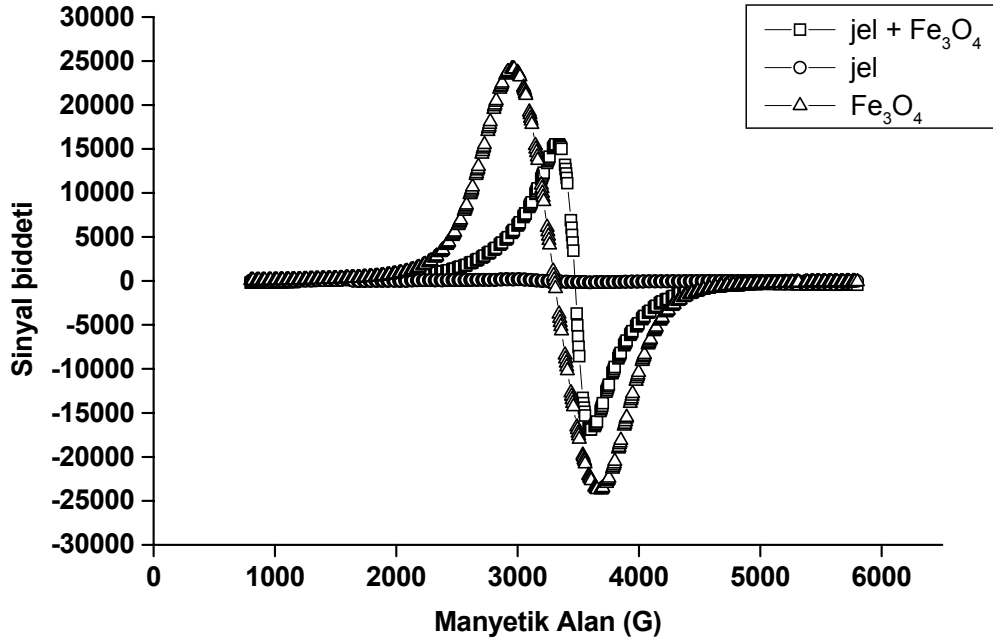
Şekil 4.9. ESR spektrumunun gösterimi: (a) Manyetik partiküller ( \text{Fe}_3\text{O}_4 ); (b) bu partikülleri içeren P(TBAAm-ko-AAm)/PVME ferrojeller; (c) manyetik olmayan P(TBAAm-ko-AAm)/PVME hidrojjeller
