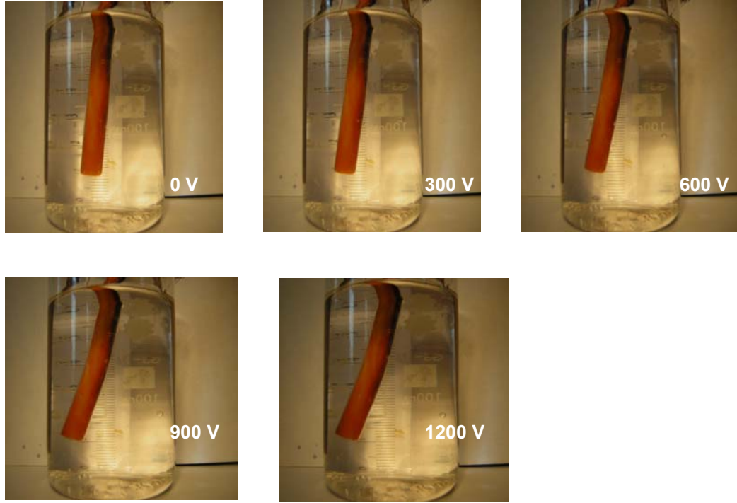
Resim 4.1. P(TBAAm-ko-AAm)/PVME ferrojellerinin elektrik alan şiddetinin bir fonksiyonu olarak katot elektrota doğru bükülmesi. Uygulanan DC voltaj arttırılmıştır (absorpsiyon yöntemi ile hazırlanmış)
