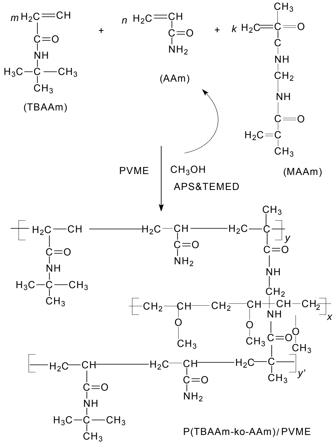
Şekil 4.2. Kimyasal yöntemle sentezlenen P(TBAAm-ko-AAm)/PVME yarı-IPN' nin olası reaksiyon mekanizması
