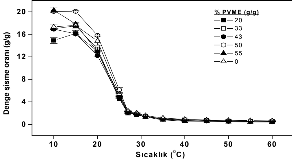
Şekil 4.3. P(TBAAm-ko-AAm)/PVME hidrojjellerinin PVME miktarına bağlı denge şişme oranı (g/g) – sıcaklık eğrisi.
