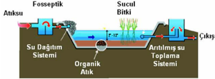
Şekil 1.1 Tipik Bir Yapay Sulak Alan Sistemi Kesiti (www.khgm.gov.tr)
