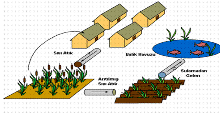
Şekil 1.3 Tipik Bir Yapay Sulak Alan Sistemi Akış Diyagramı (www.khgm.gov.tr)
