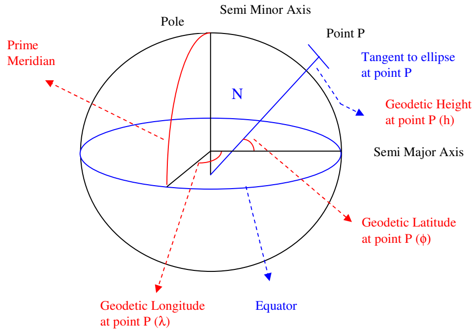
Figure 5.6. Geodetic latitude, longitude and height
