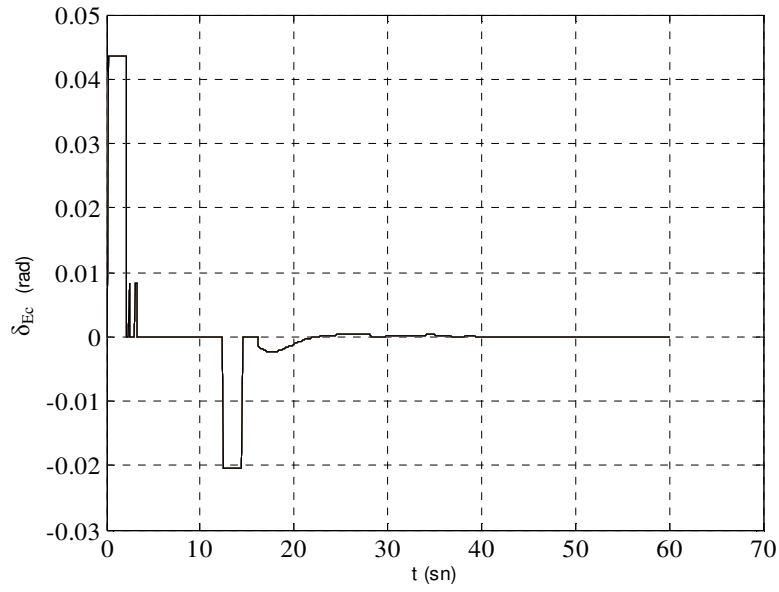
Şekil 10. Örnek 2 için irtifa dümeni açısının zamana göre değişimi (tüm jenerasyonlar)
