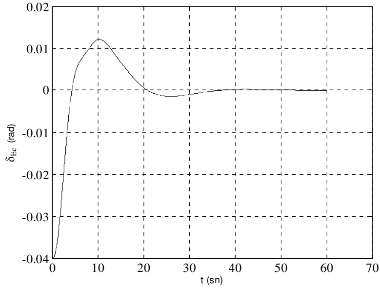
Şekil 4.5. İrtifa dümeni açısının zamana göre değişimi (1.uçuş durumu K_p=-0.0008 ve K_d=-0.0005 )
