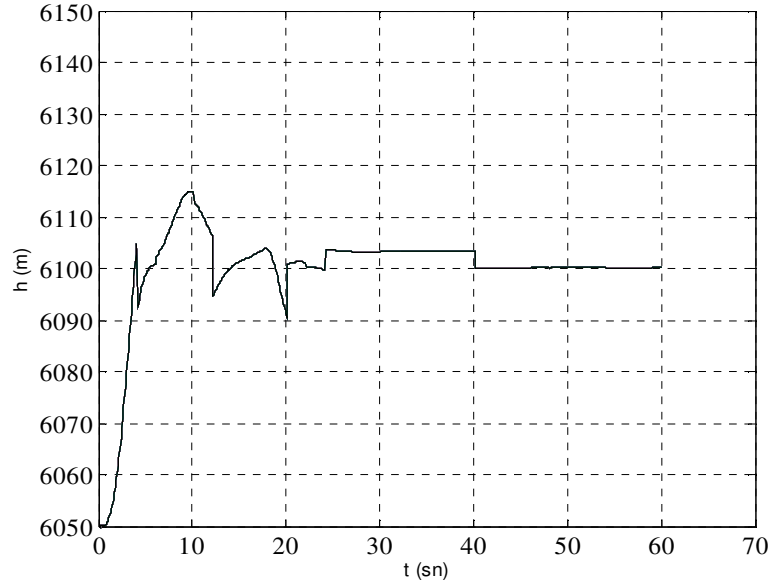
Şekil 4.30. Örnek 1 için irtifanın zamana göre değişimi (tüm jenerasyonlar)
