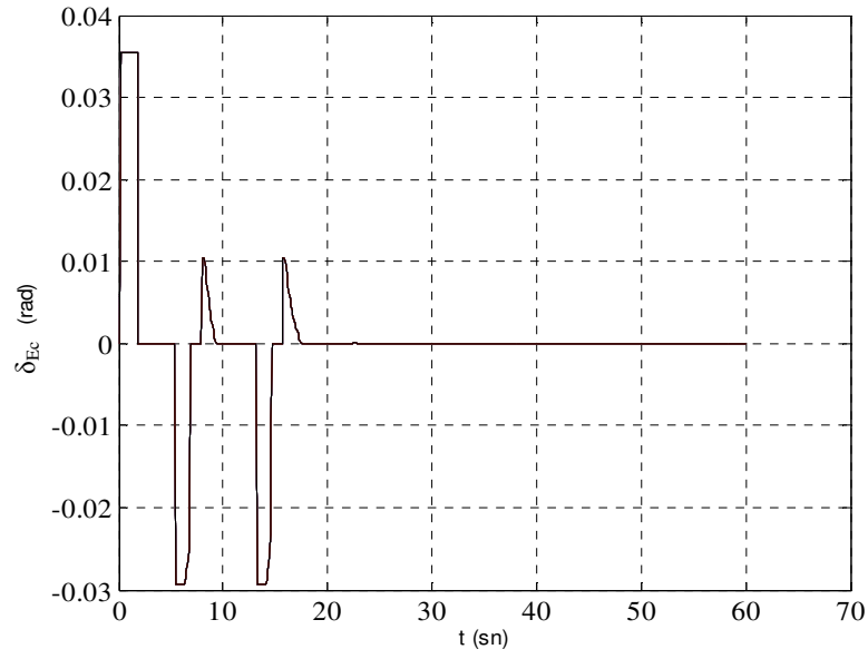
Şekil 46. Örnek 6 için irtifa dümeni açısının zamana göre değişimi (son jenerasyondaki en iyi dizi)
