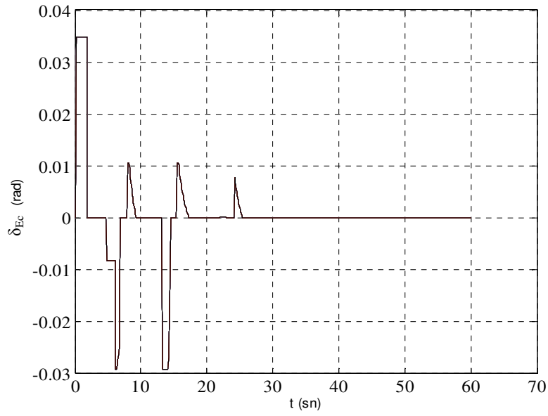
Şekil 42. Örnek 6 için irtifa dümeni açısının zamana göre değişimi (tüm jenerasyonlar)
