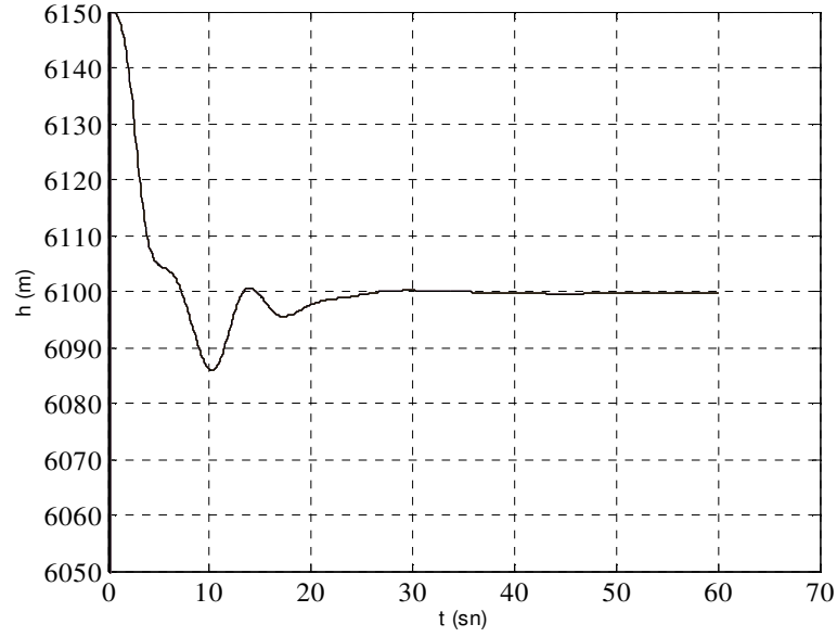
Şekil 15. Örnek 2 için irtifanın zamana göre değişimi (son jenerasyondaki en iyi dizi)
