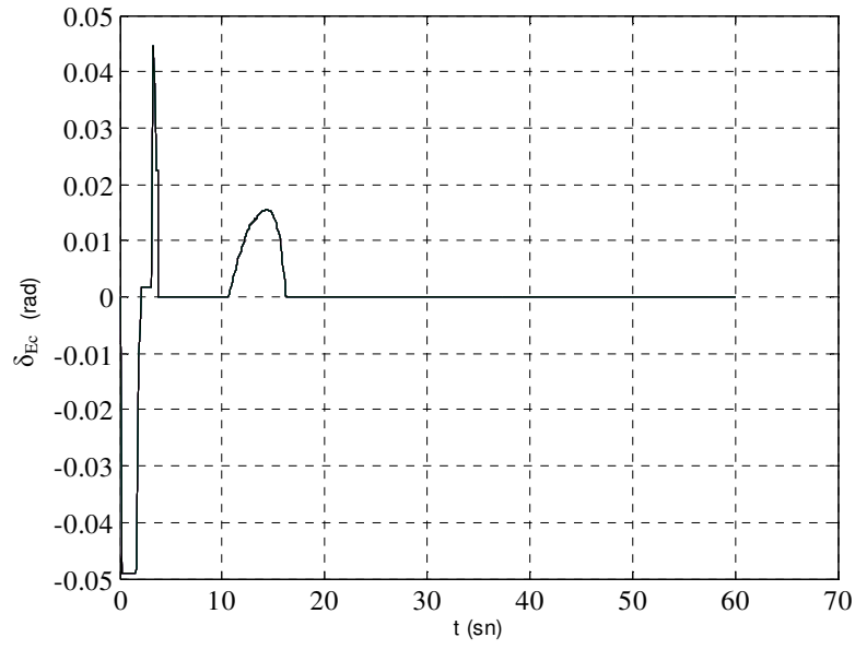
Şekil 4.33. Örnek 1 için irtifa dümeni açısının zamana göre değişimi (son jenerasyondaki en iyi dizi)
